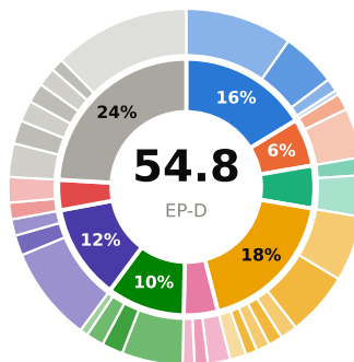
kNN baseline
