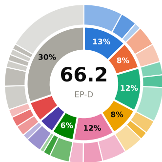
Gemini-3.1-Pro
