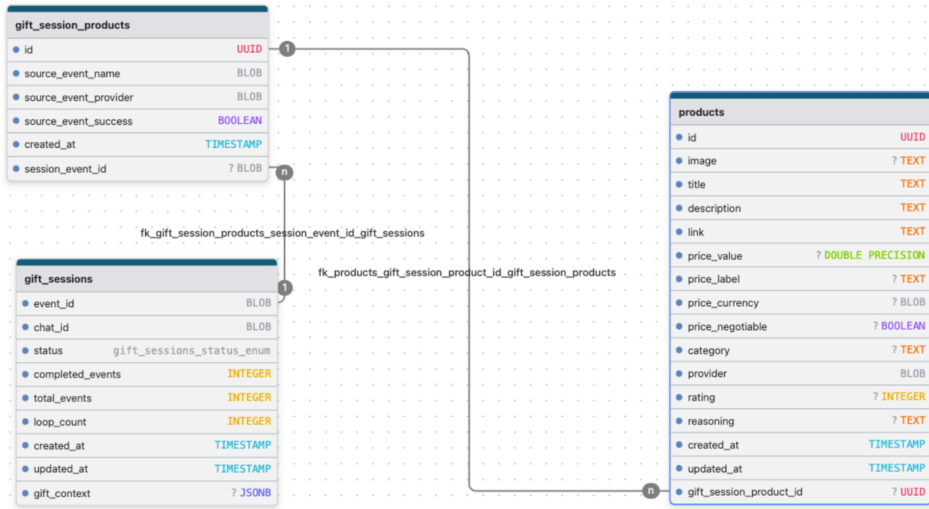
Rysunek 15: Schemat bazy danych mikroserwisu Reranking .
