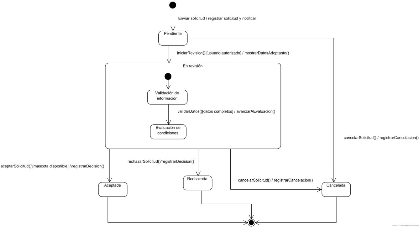
Anexo C.7: Diagrama de Máquina de Estados UML — Entidad SolicitudAdopcion
