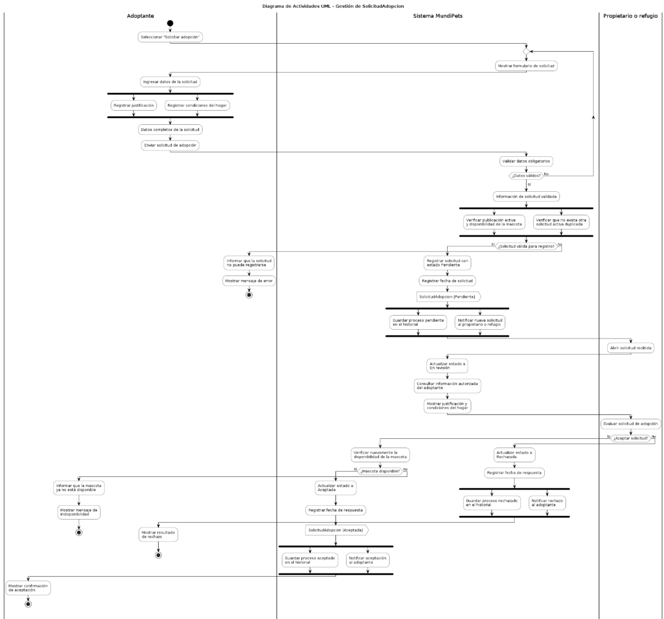
Anexo C.6: Diagrama de Actividades UML — Gestión de Solicitud de Adopción (RF-05)
