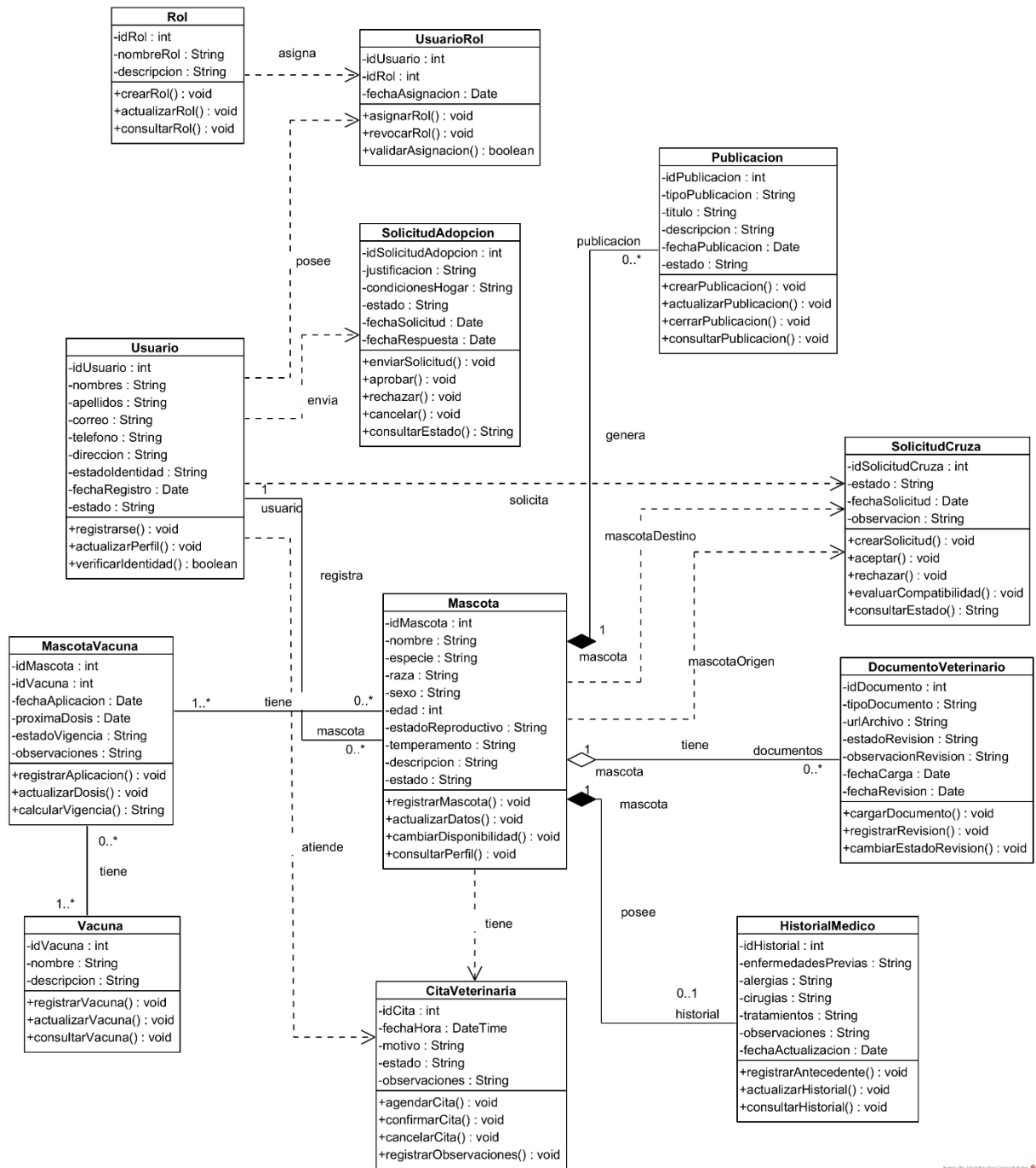
Anexo C.2: Diagrama de Clases UML — Sistema MundiPets
