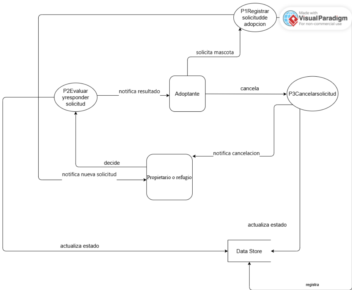
Anexo C.5: DFD Esencial — Proceso de Gestión de Solicitudes de Adopción
