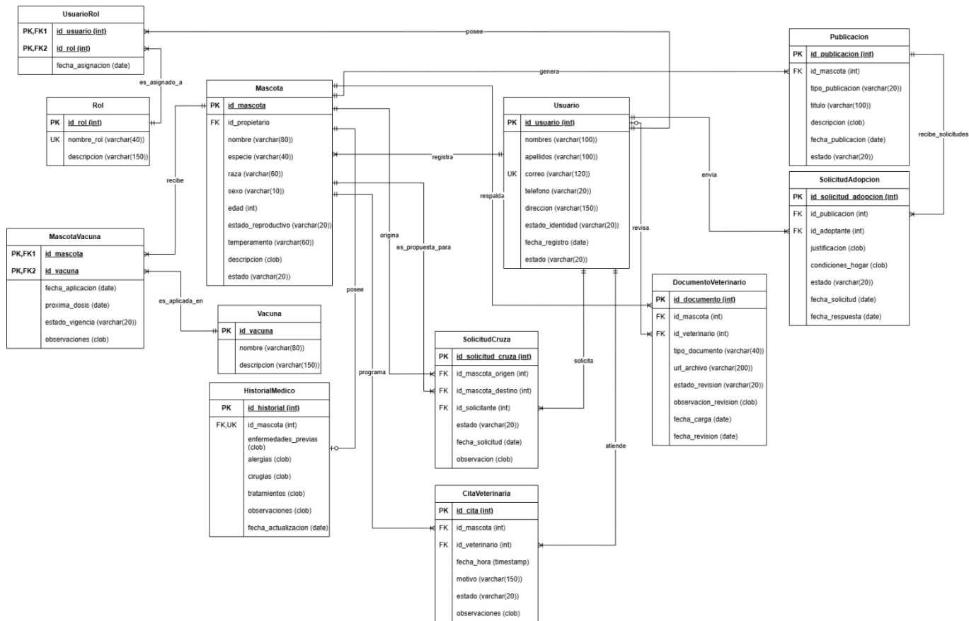
Anexo C.1: Diagrama Entidad-Relación del Modelo de Datos — Sistema MundiPets
