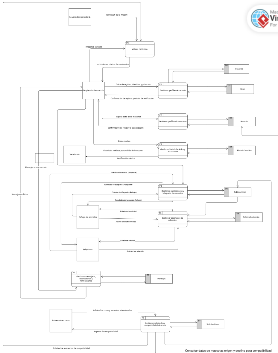
Anexo C.4: DFD Nivel 1 — Descomposición de Procesos del Sistema MundiPets
