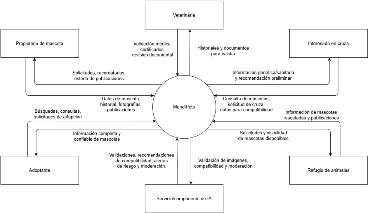
Anexo C.3: DFD Nivel 0 — Diagrama de Contexto del Sistema MundiPets
