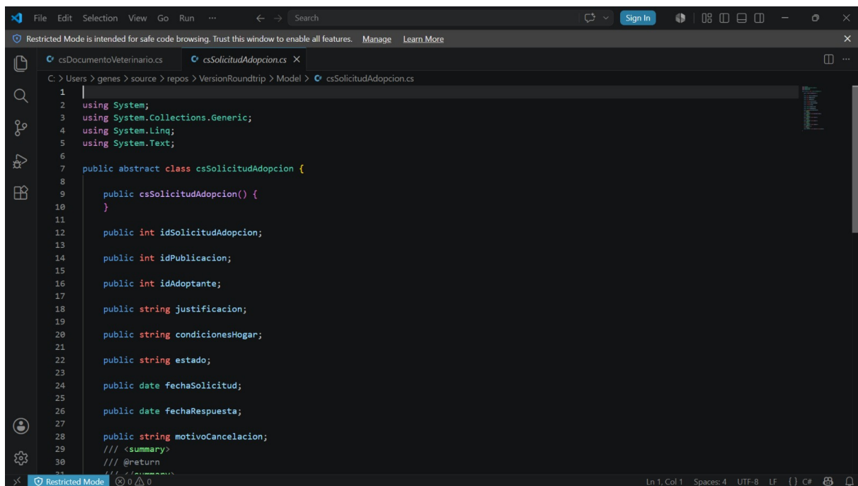
Figura 29: Código generado — csSolicitudAdopcion.cs
