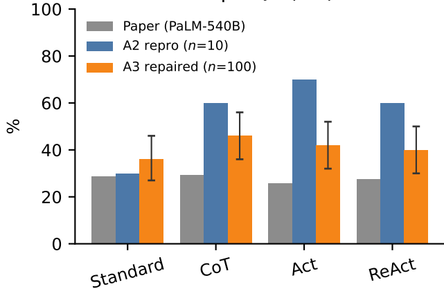
HotpotQA (EM)
