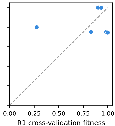
SpeciAL (MAE 0.209)
