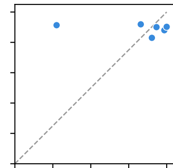
SpeciAL (MAE 0.209)
