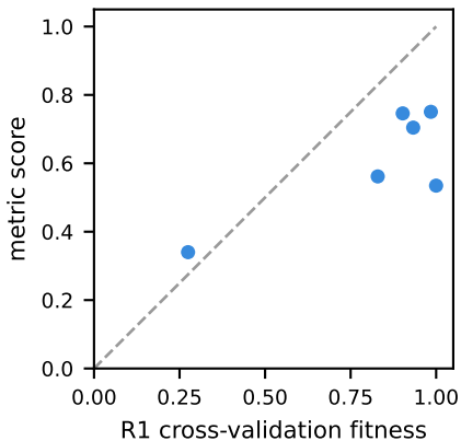
AVATAR (MAE 0.236)
