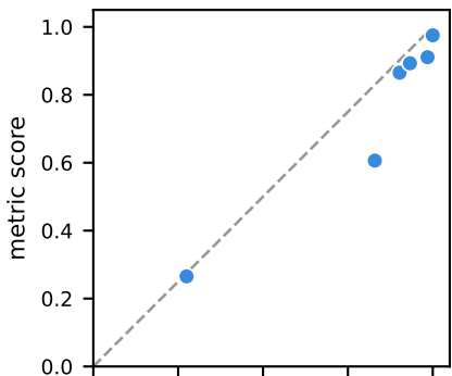
AVATAR (MAE 0.236)
