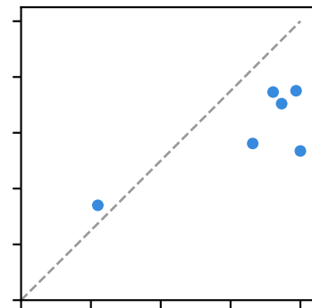
SpeciAL (MAE 0.209)
