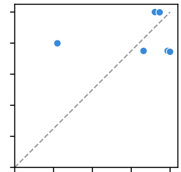
SpeciAL (MAE 0.209)
