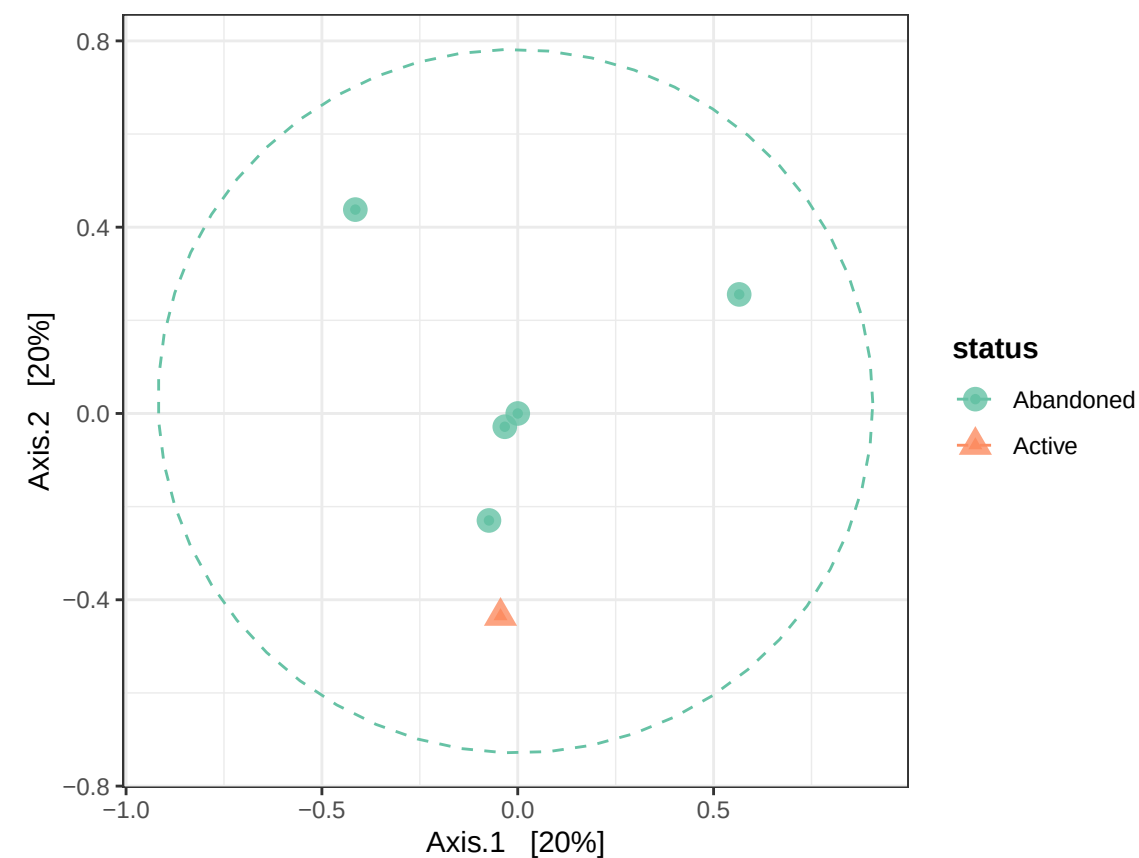
Diversité Bêta (PCoA – Bray–Curtis)
