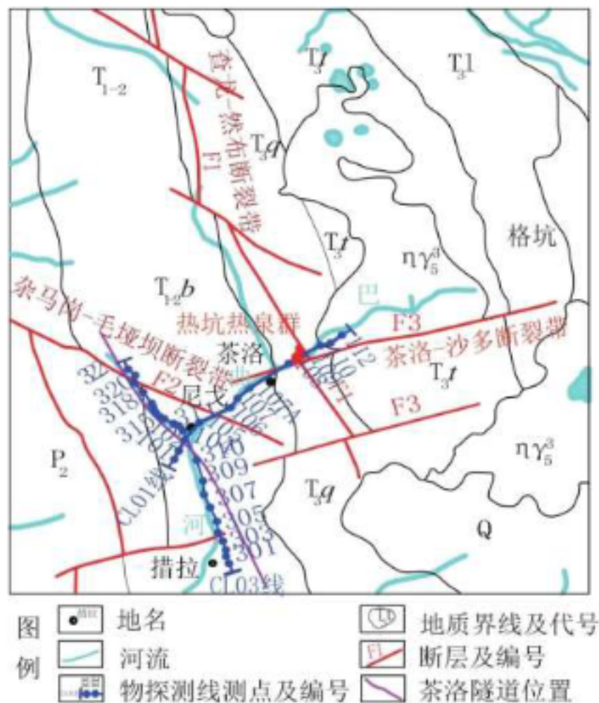
(b) 研究区地质简图
