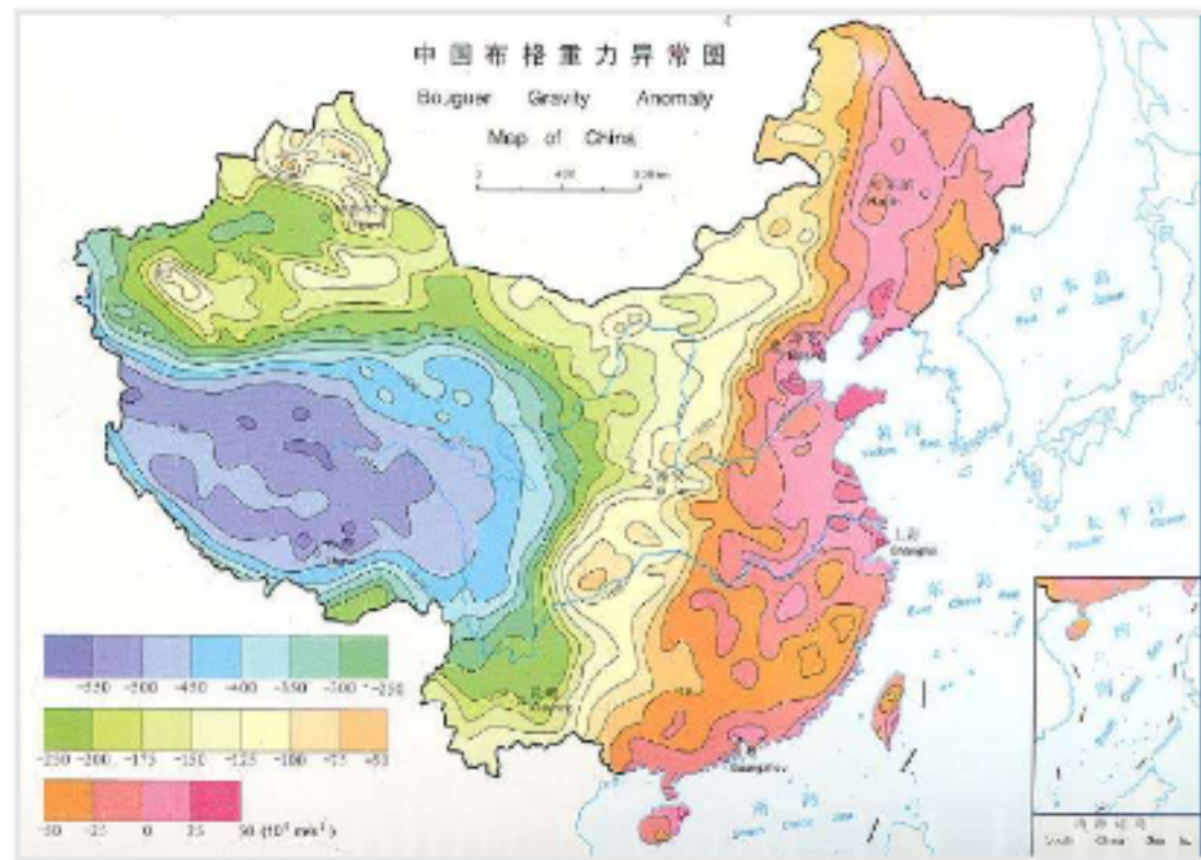
中国布格重力异常图
