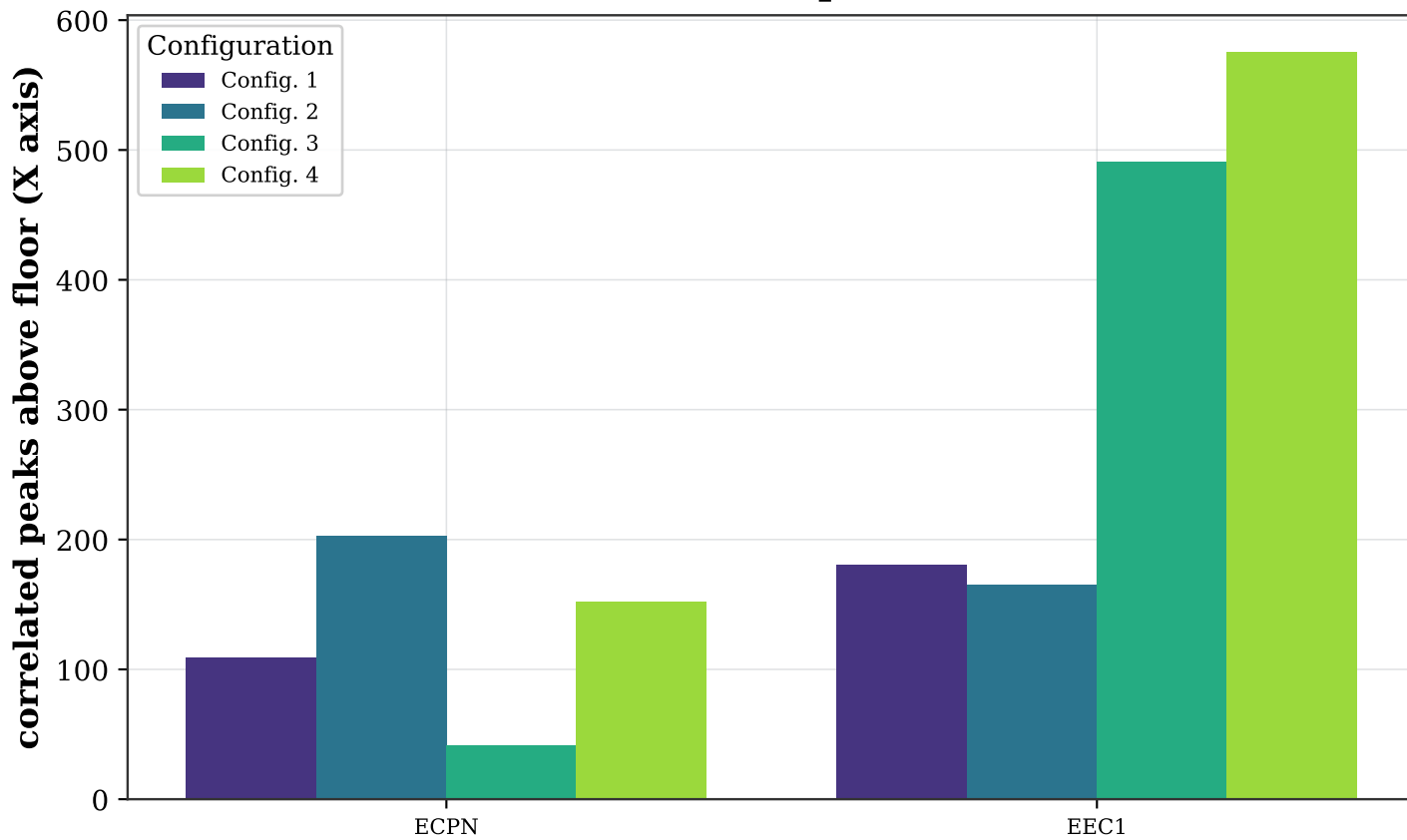
INGV (eruptive)
