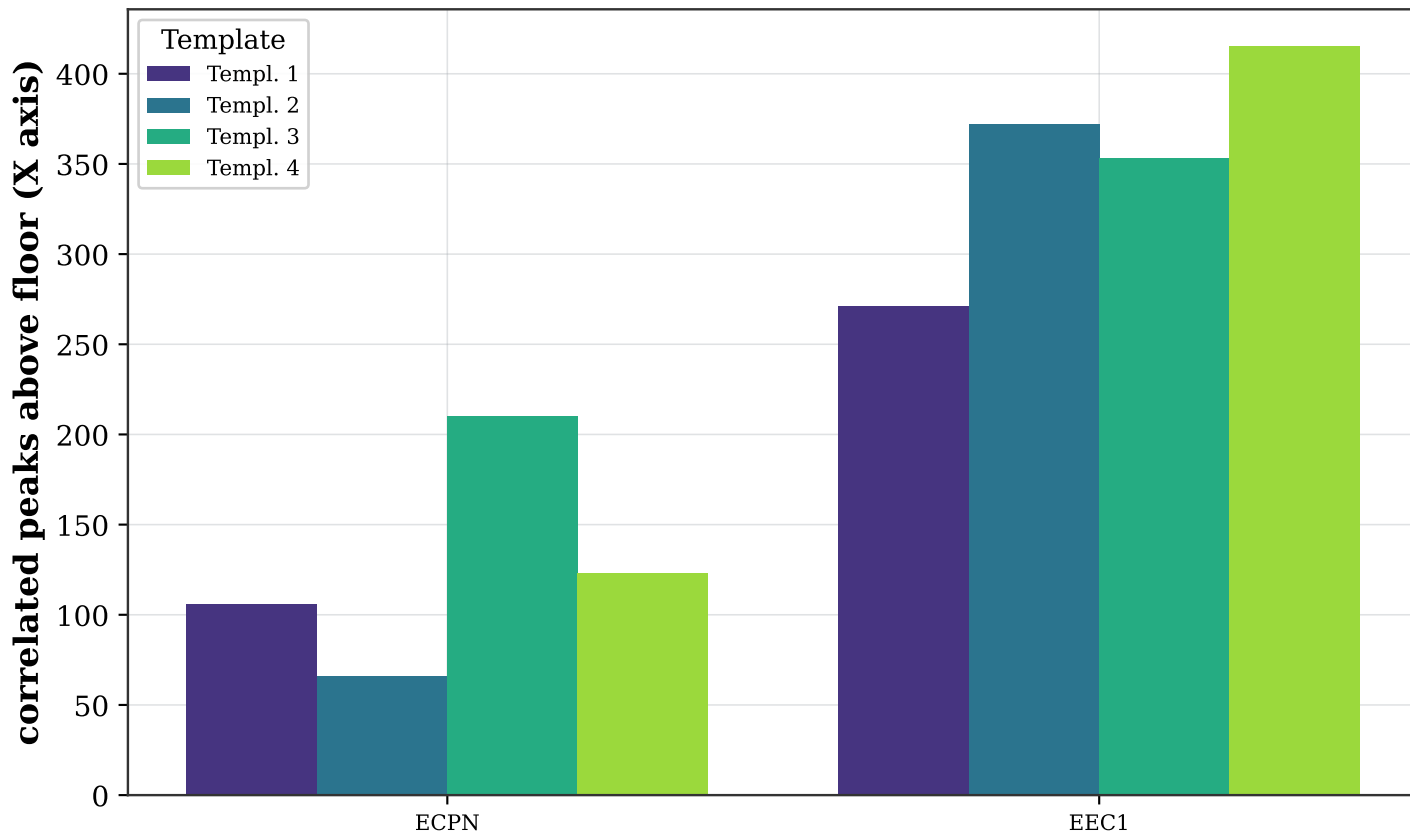
INGV (eruptive)
