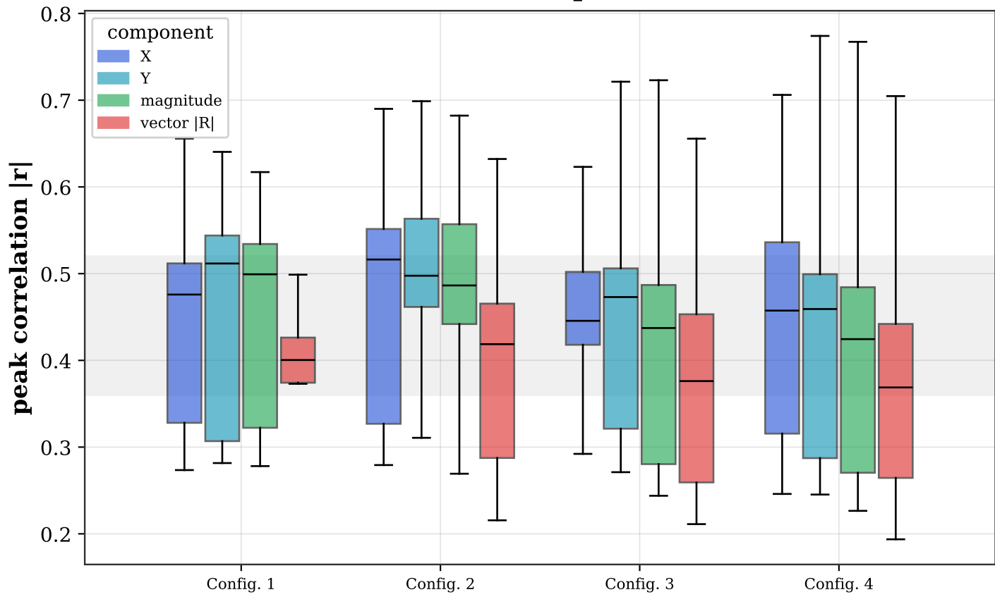
INGV (eruptive)
