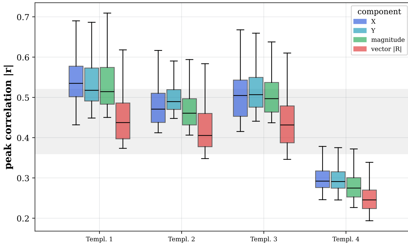
INGV (eruptive)
