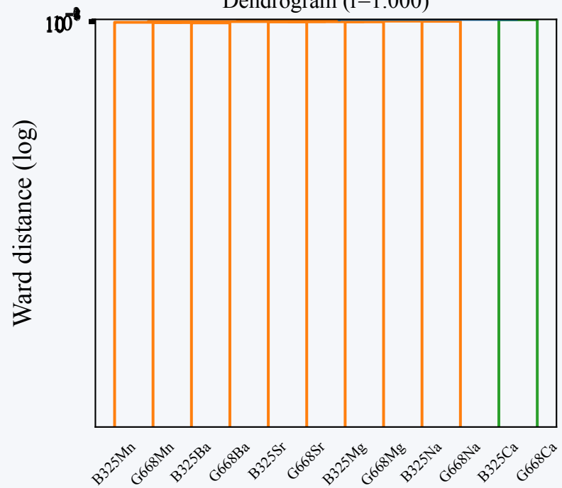
Dendrogram (r=1.000)
