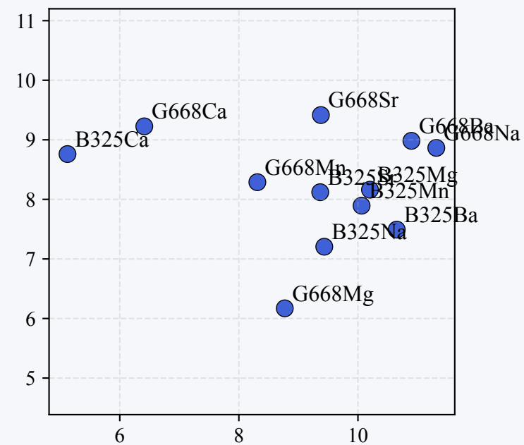
UMAP
