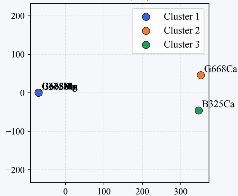
K-Means (k=3)
