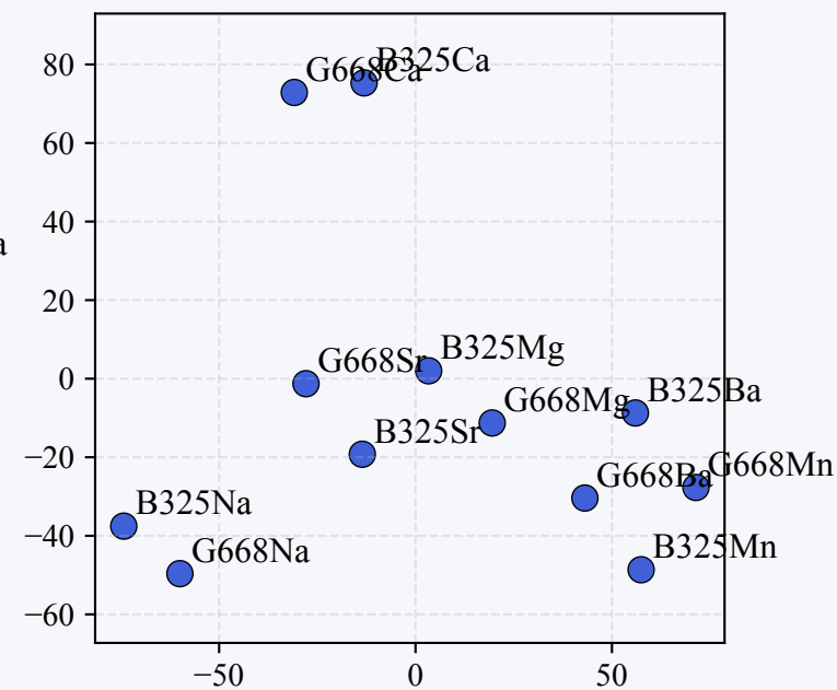
t-SNE
