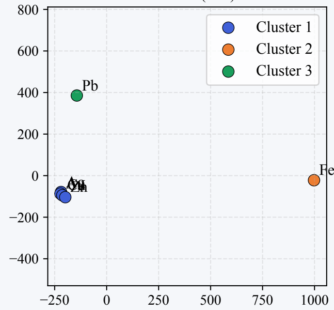
K-Means (k=3)
