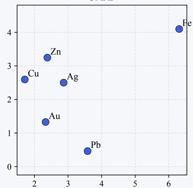
UMAP
