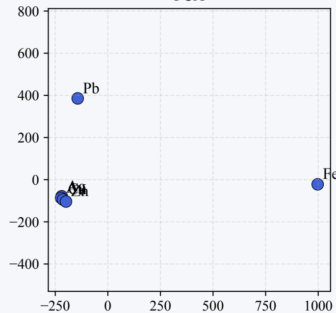
PCA
