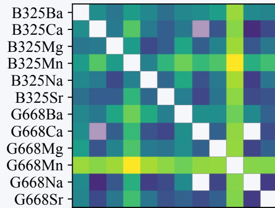
Cosine
