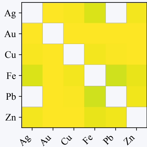
Cosine
