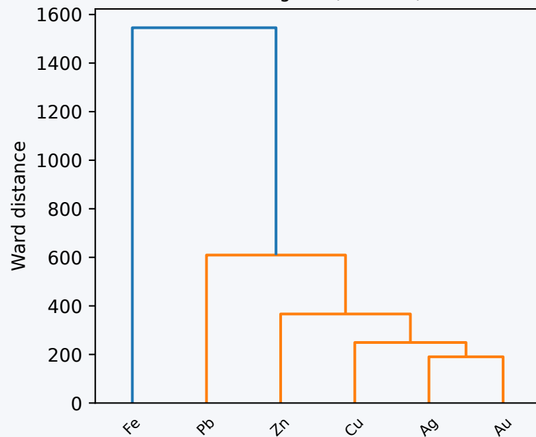
Dendrogram (r=1.000)
