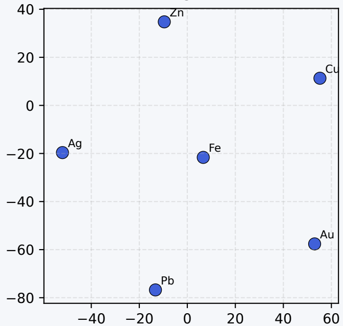
t-SNE
