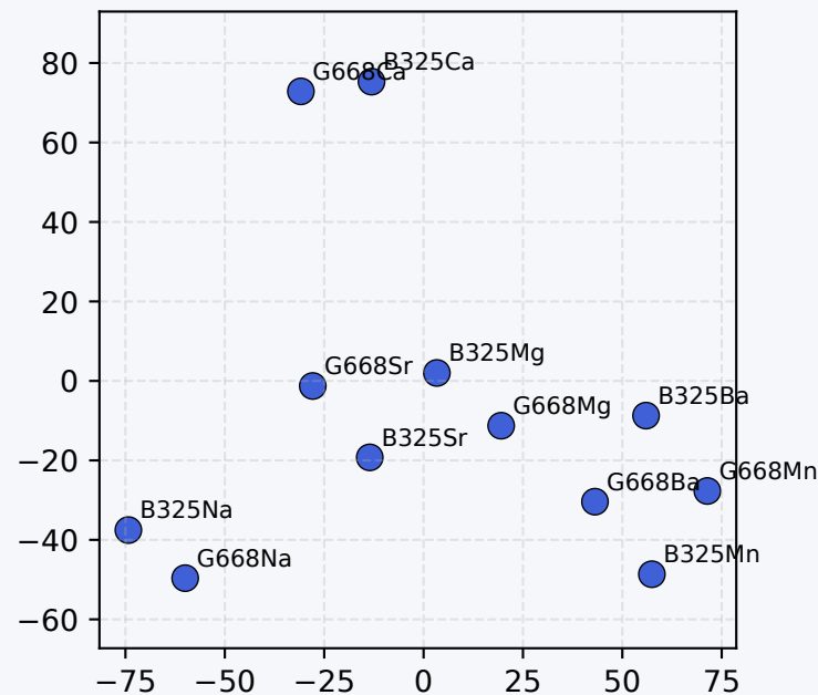
t-SNE
