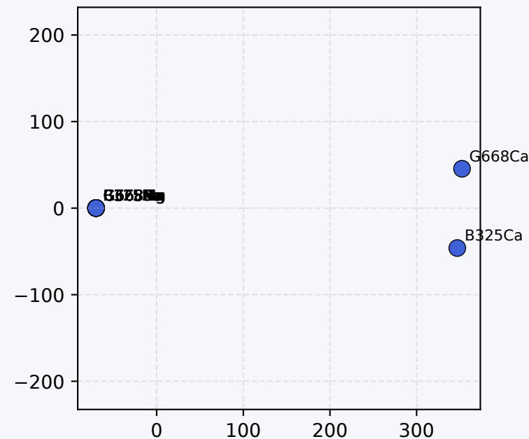
PCA
