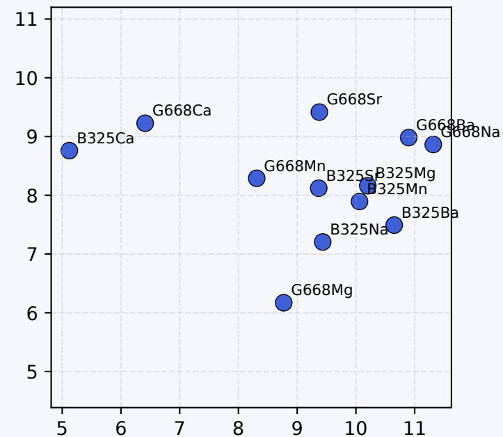
UMAP
