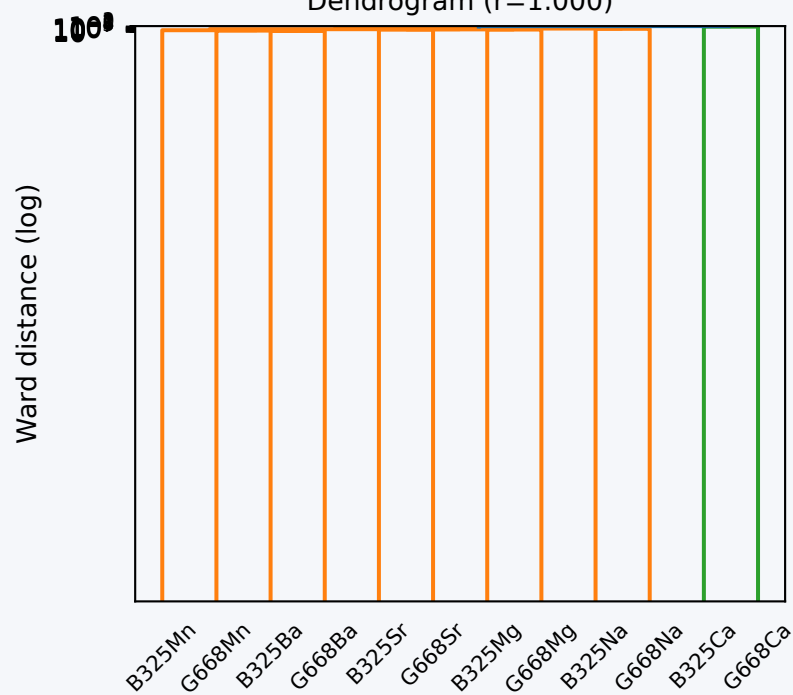
Dendrogram (r=1.000)
