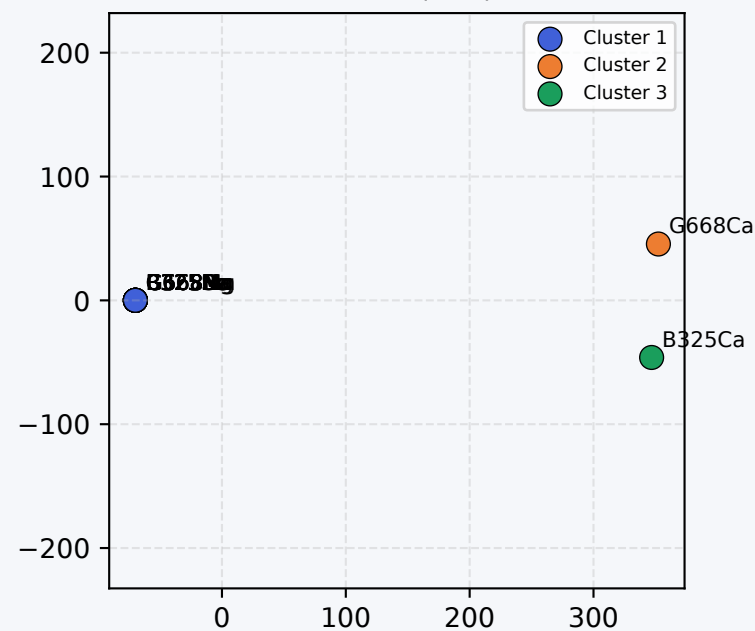
K-Means (k=3)
