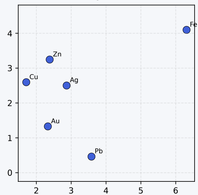
UMAP
