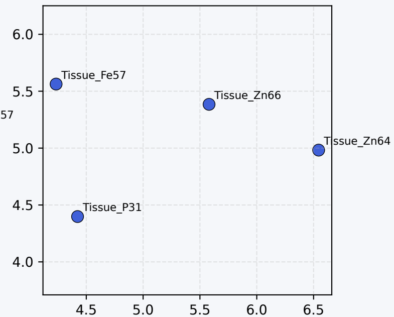
UMAP
