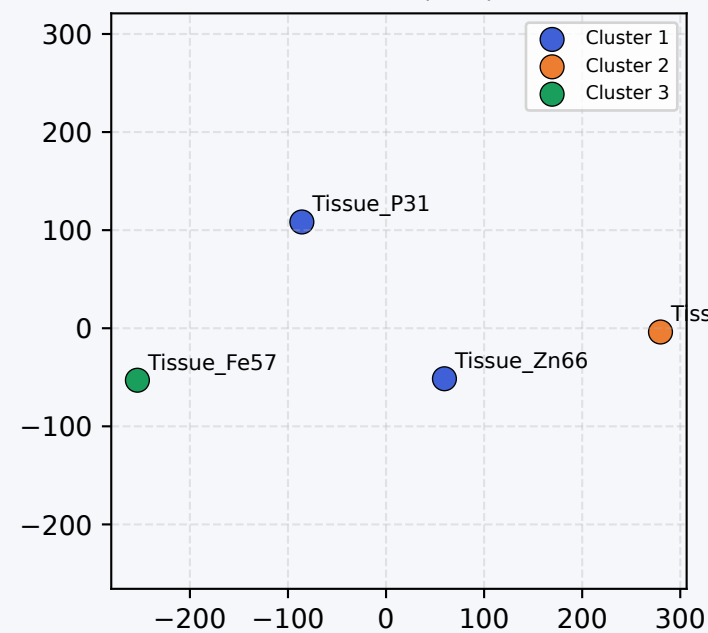
K-Means (k=3)
