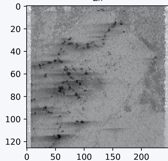
Zn
