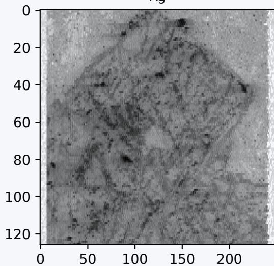
Fe
