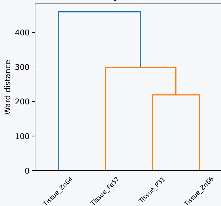
Dendrogram (r=0.597)
