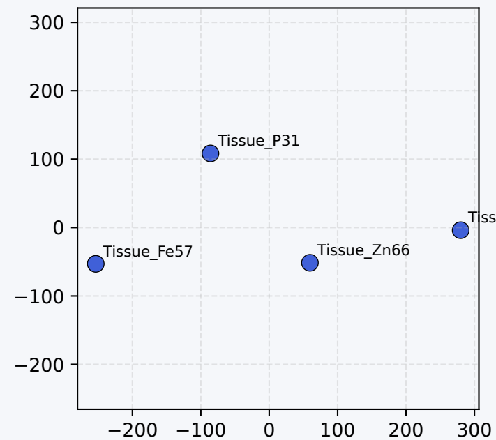
PCA
