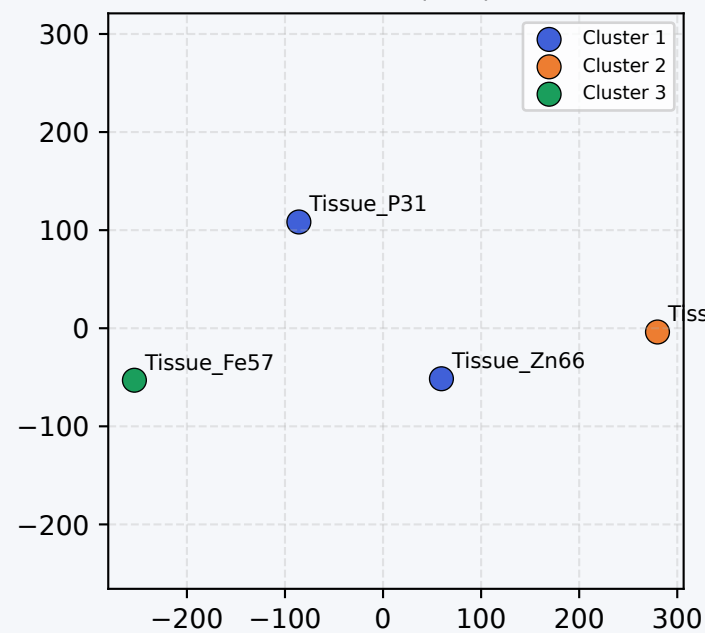
K-Means (k=3)
