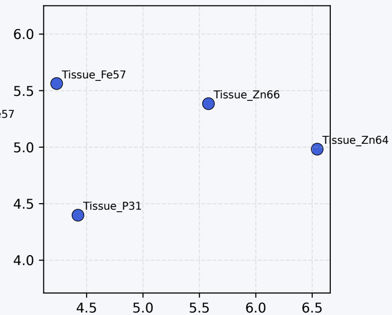
UMAP
