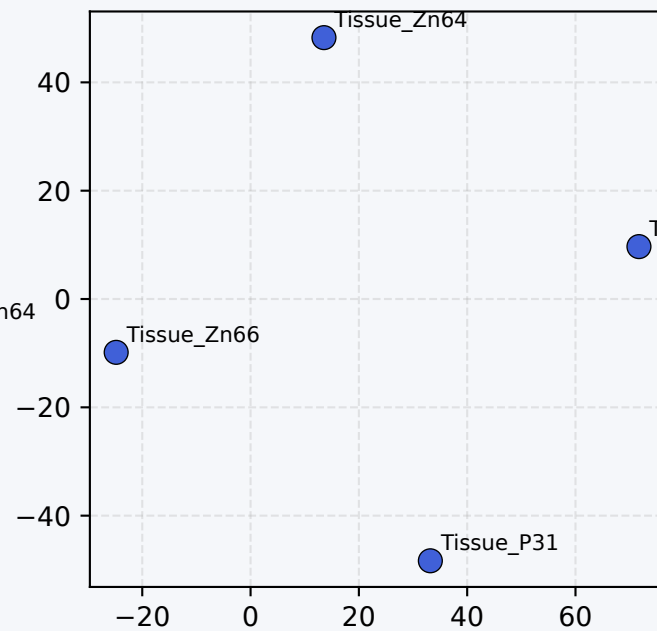
t-SNE
