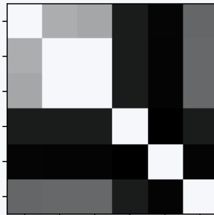
Minkowski
