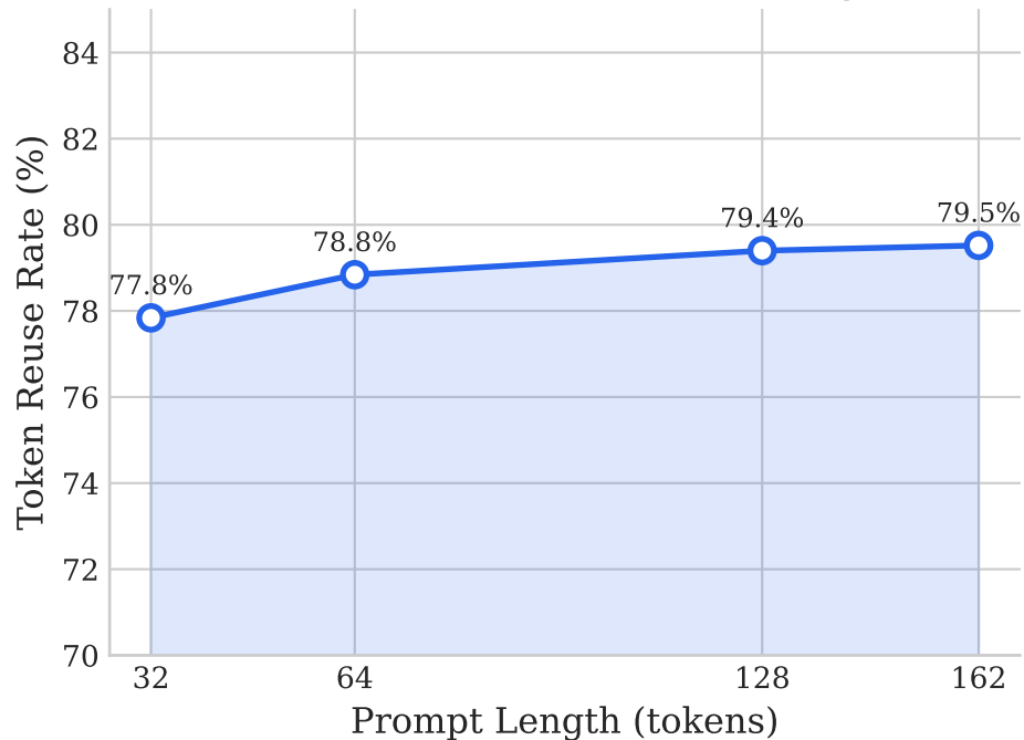
(a) Token Reuse vs Prompt Length
