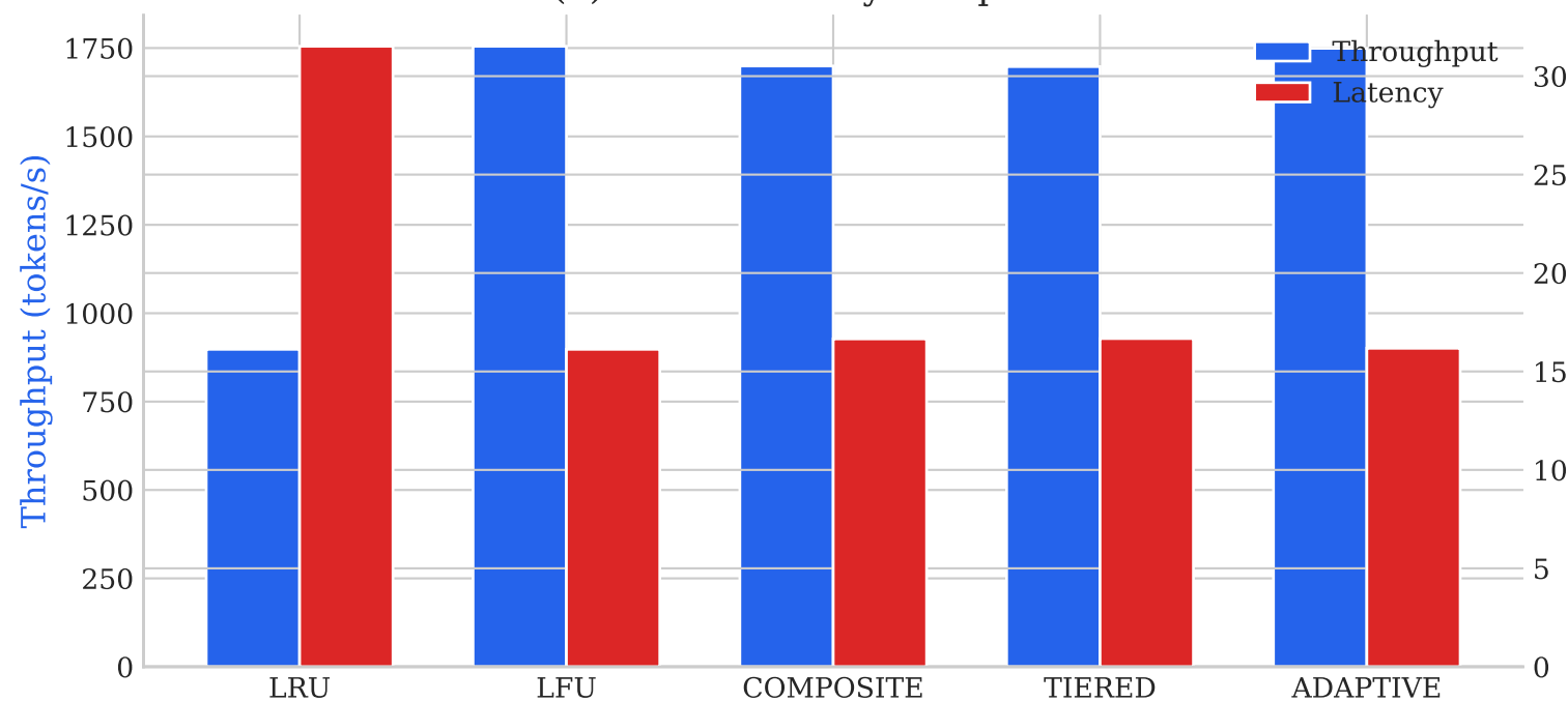
(d) Eviction Policy Comparison
