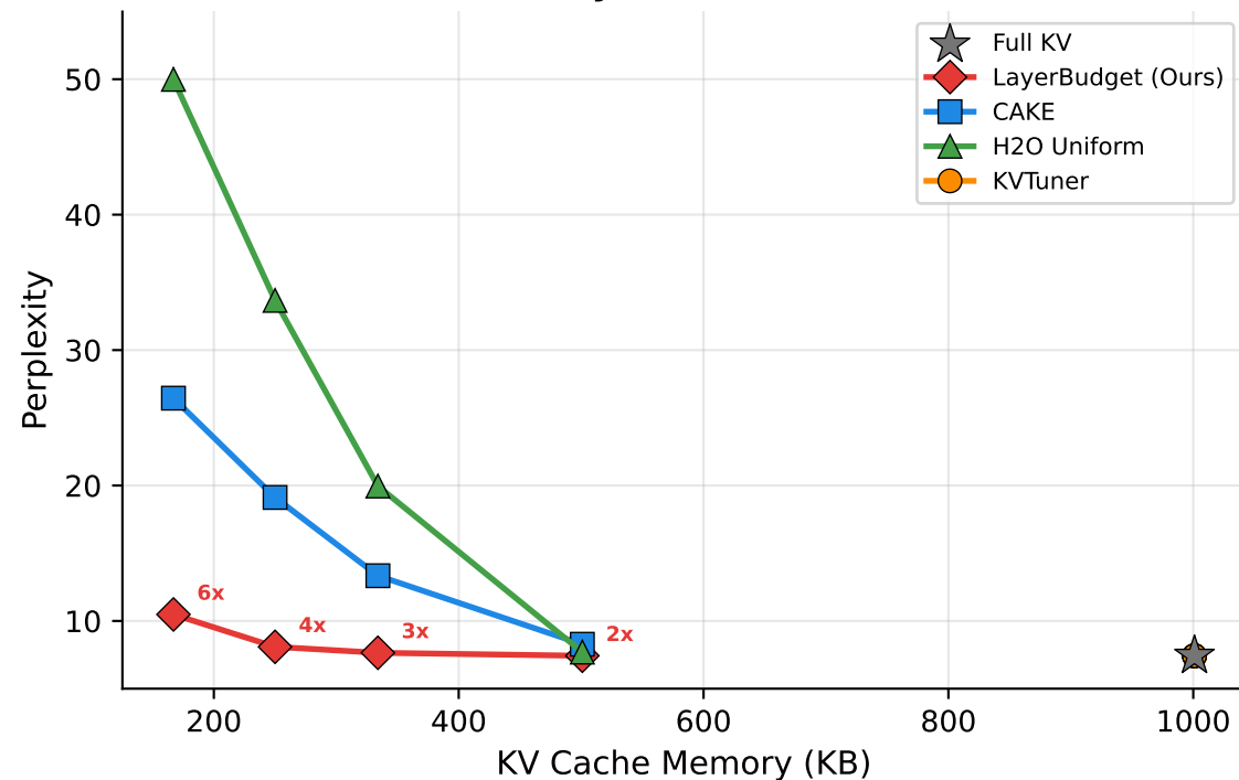
TinyLlama-1.1B
