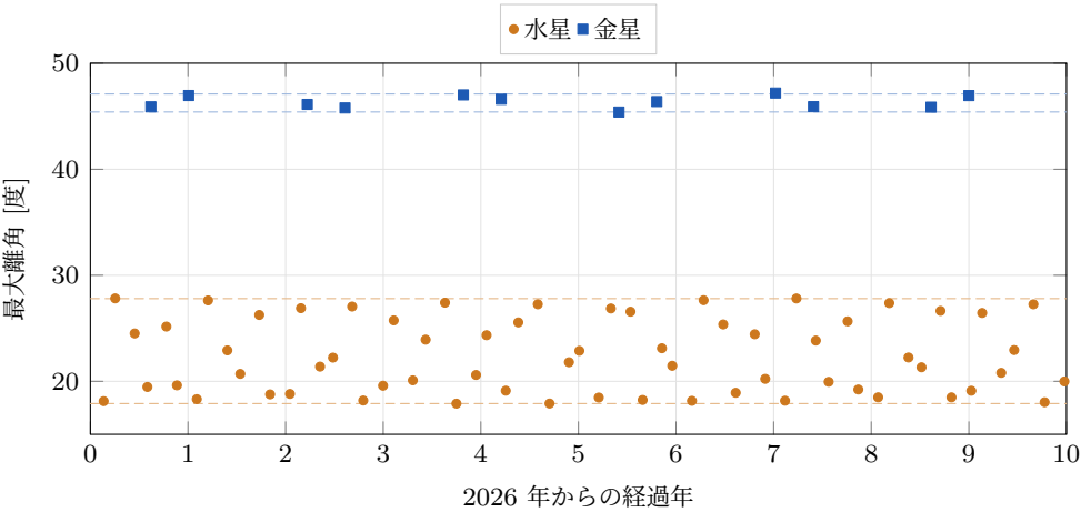
図 6 2026 年から 10 年間に起こる最大離角の分布。破線は天文年鑑等で知られる変動範囲（水星 17.9°–27.8°、金星 45.4°–47.1°）。離心率が 0.206 と大きい水星は、最大離角がどの位置で起こるかによって 10° 近く変動する。一方、金星の軌道はほぼ円（ e = 0.0068 ）なので、最大離角は 46° 前後にきれいに集中する。
