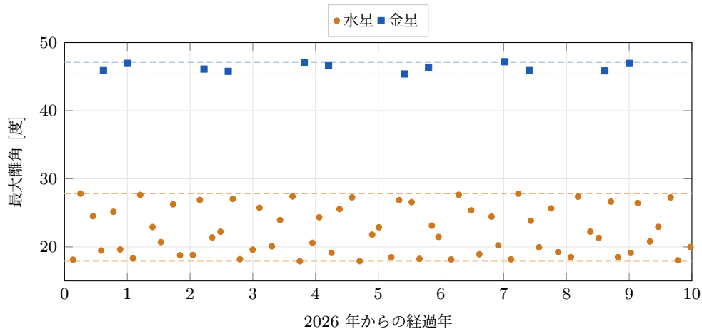
図6 2026年から10年間に起こる最大離角の分布。破線は天文年鑑等で知られる変動範囲（水星 17.9^{\circ} – 27.8^{\circ} 、金星 45.4^{\circ} – 47.1^{\circ} ）。離心率が0.206と大きい水星は、最大離角がどの位置で起こるかによって 10^{\circ} 近く変動する。一方、金星の軌道はほぼ円（ e = 0.0068 ）なので、最大離角は 46^{\circ} 前後にきれいに集中する。
