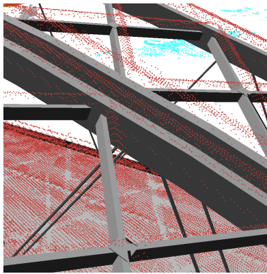
Figuur 54 AHN4 (rood) vergeleken met het IFC model (grijs)
