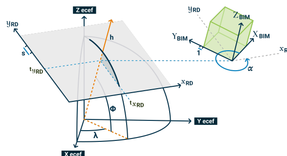
Figuur 10 2D Transformatie + 1D Transformatie
