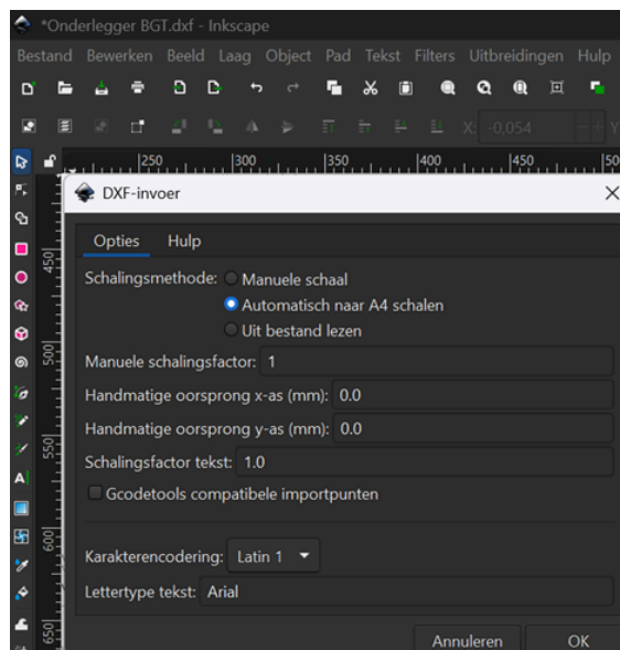
Figuur 33 Importeren van DXF-onderlegger in Inkscape.
