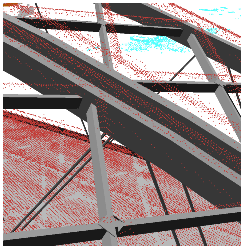
Figuur 46 AHN4 (rood) vergeleken met het IFC model (grijs)
