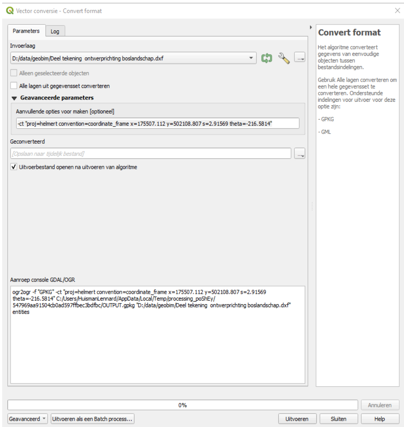
Figuur 40 QGIS Vector Conversie
