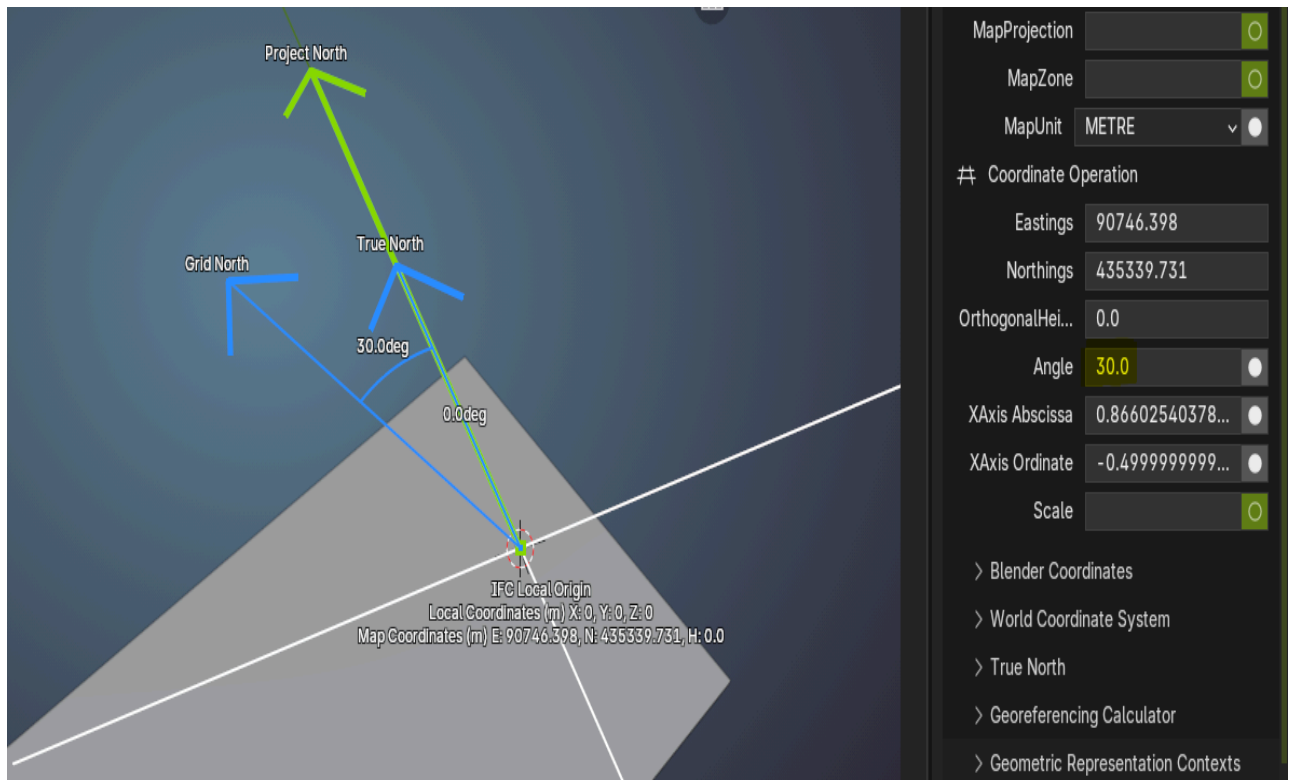
Figuur 31 Georeferentie van IFC bekijken in Blender
