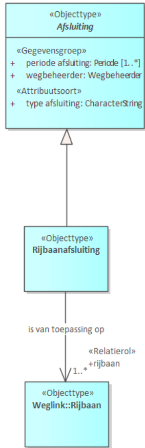
Figuur 39 – Diagram: Rijbaanafsluiting
