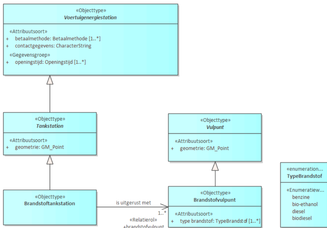
Figuur 21 – Diagram: Brandstoftankstation
