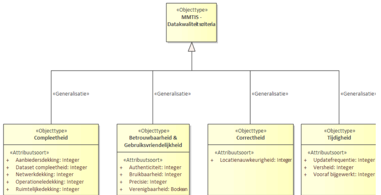
Figuur 74 – Diagram: MMTIS - Datakwaliteit
