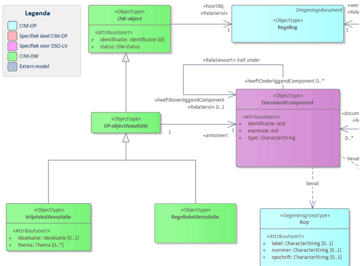
Figuur 11 DocumentComponenten
