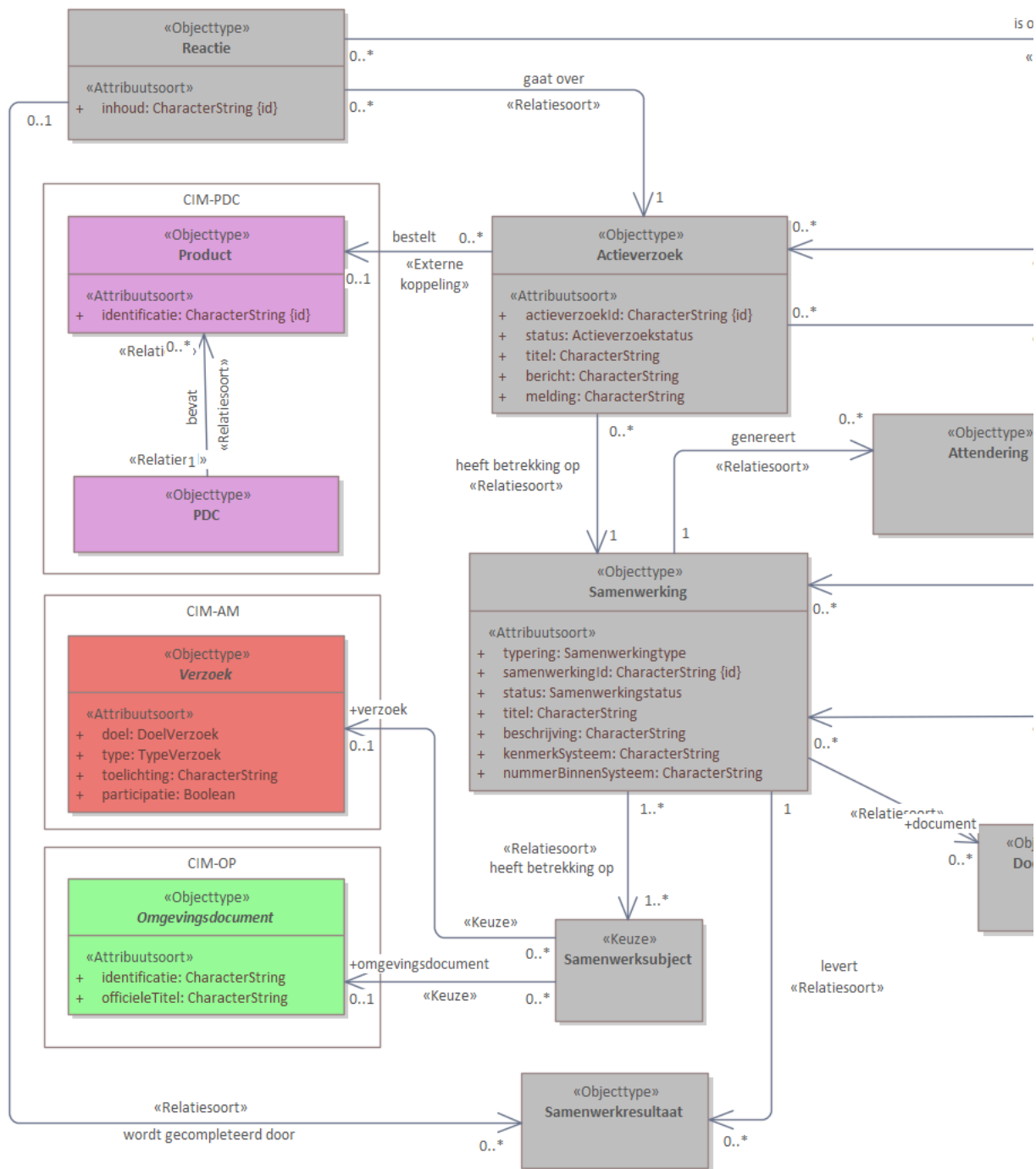
Figuur 3 – Diagram: CIM-SWF
