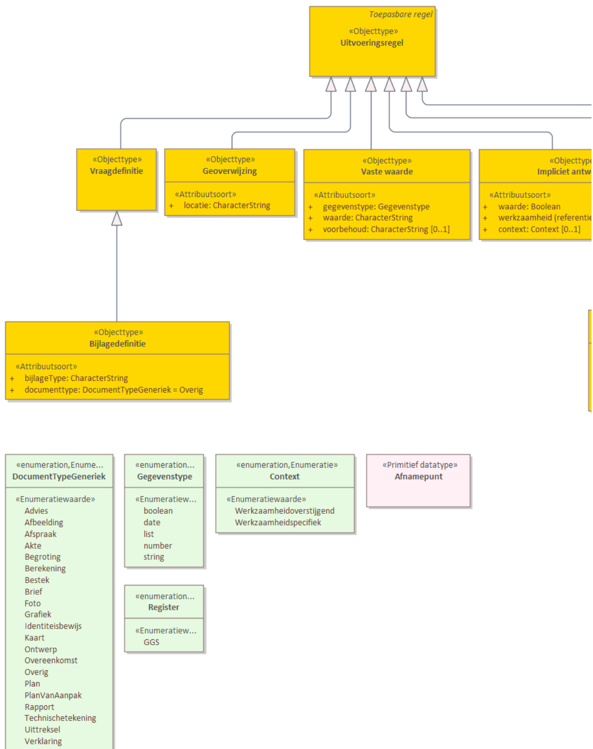
Figuur 5 – Diagram: CIM-TR Uitvoeringsregels
