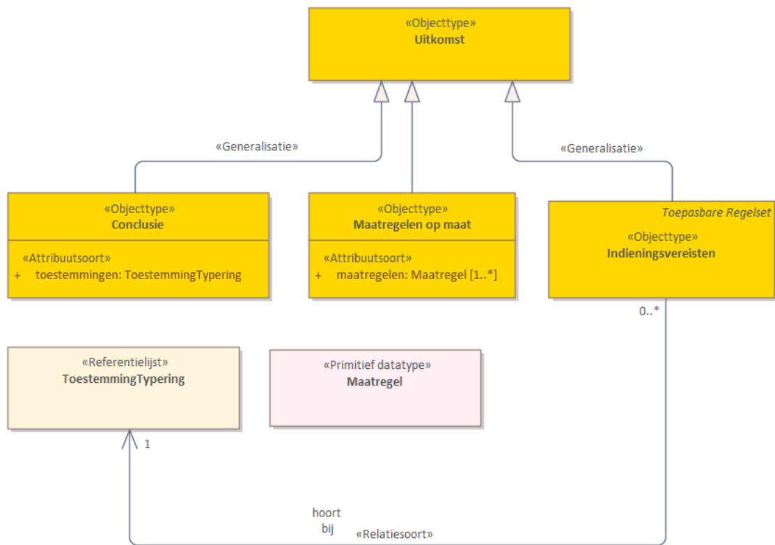
Figuur 4 – Diagram: CIM-TR Uitkomsten
