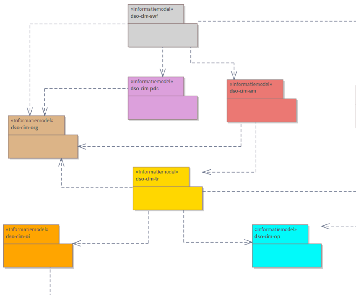
Figuur 2 – Diagram: CIM-TR Context
