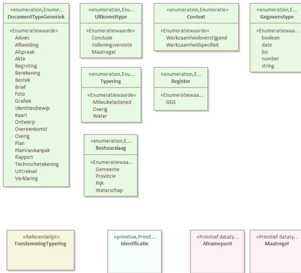
Figuur 10 – Diagram: CIM-TR Datatypen en waardelijsten
