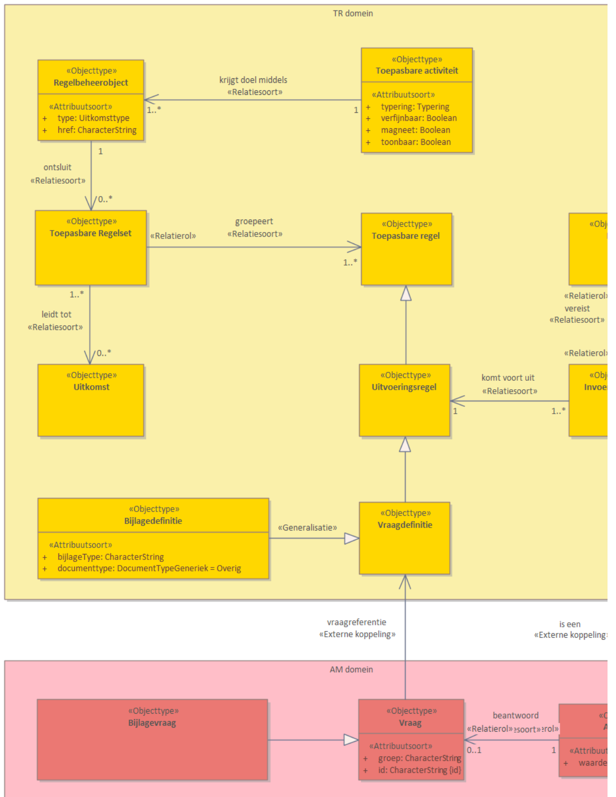
Figuur 9 – Diagram: CIM-TR Opstellen aanvraag
