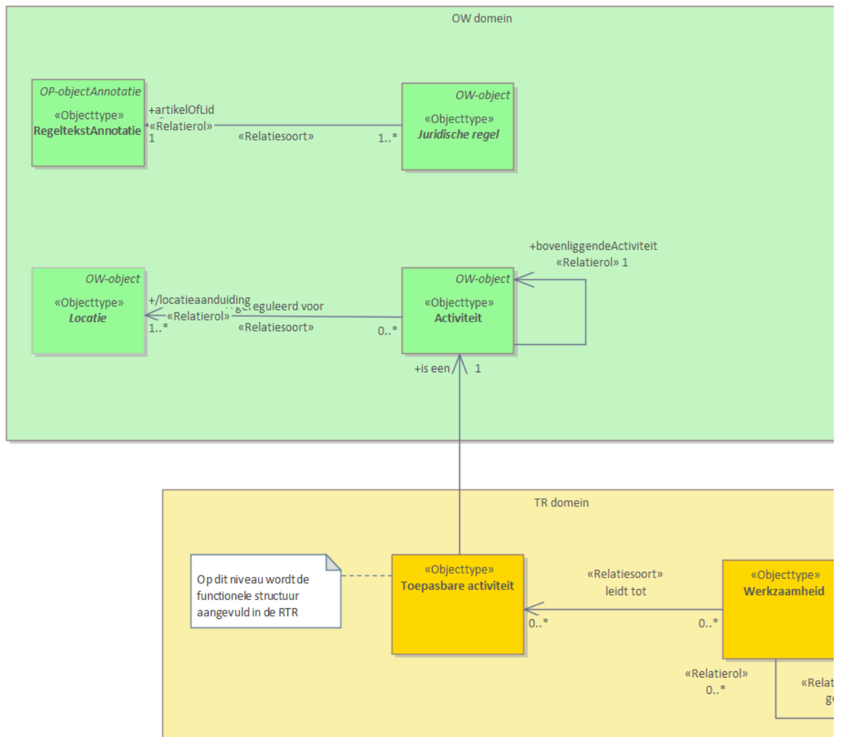
Figuur 6 – Diagram: CIM-TR Functionele Structuur
