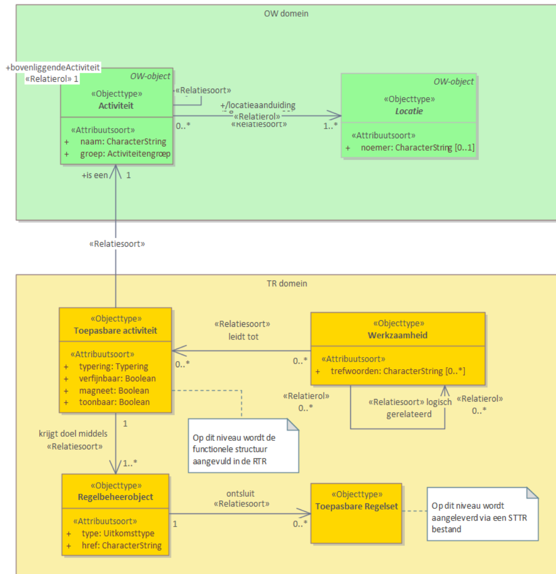
Figuur 7 – Diagram: CIM-TR Toepasbare Activiteit
