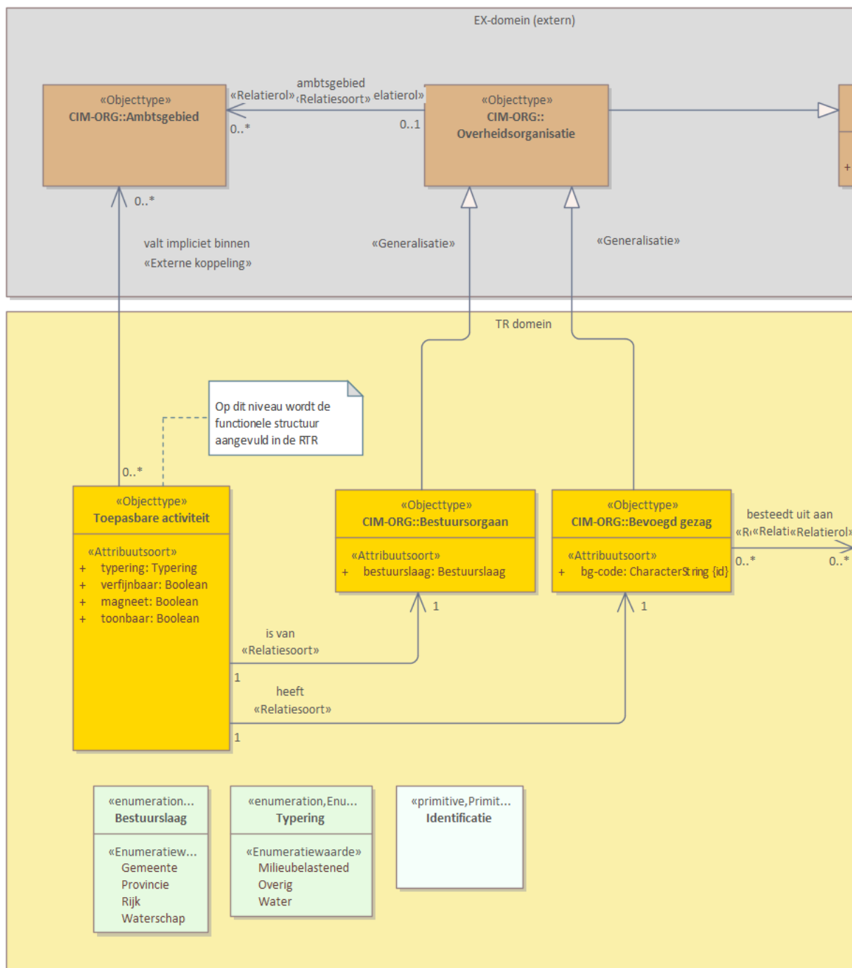
Figuur 8 – Diagram: CIM-TR Behandeldienstconfiguratie
