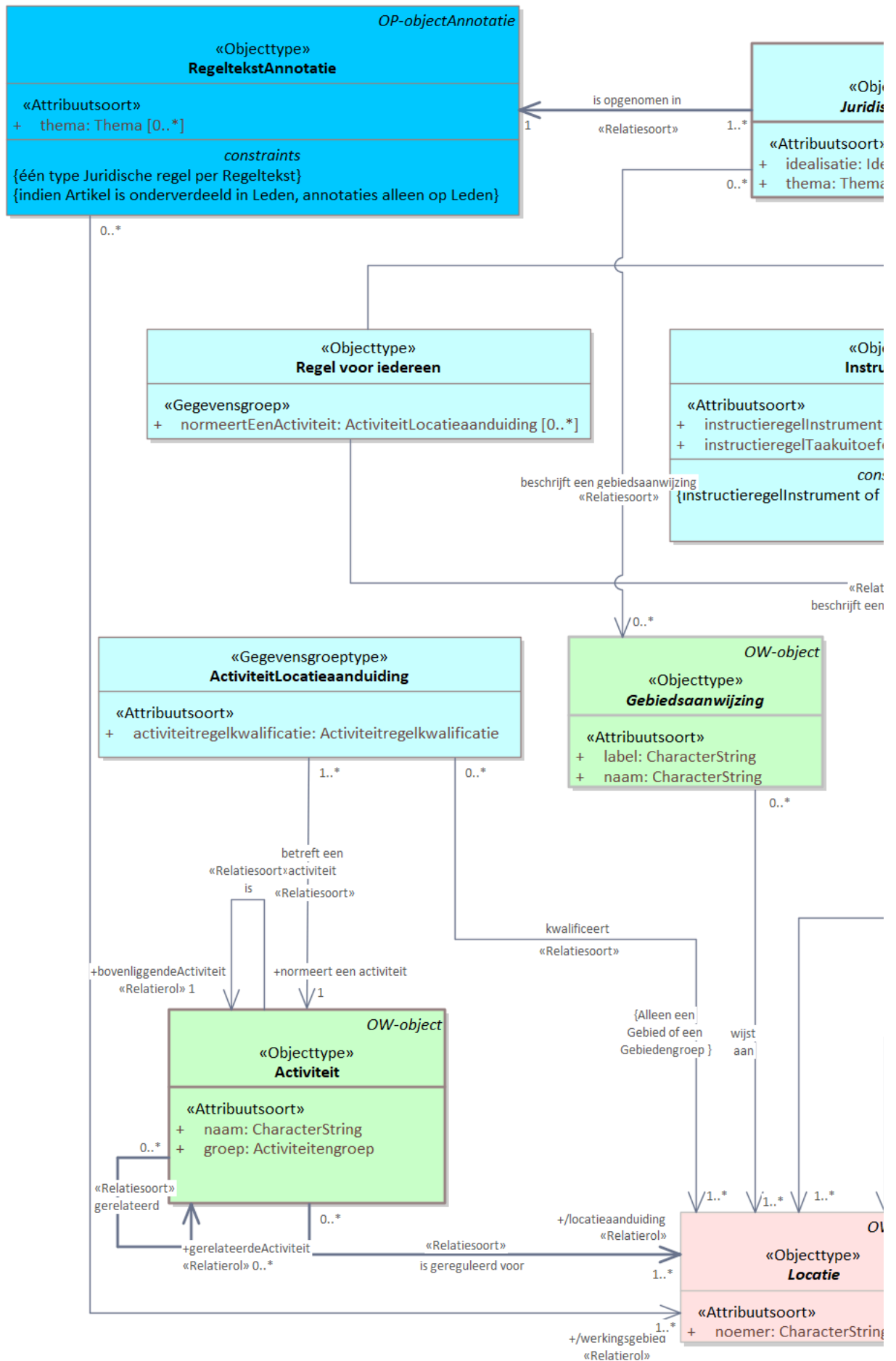
Figuur 11 Regels voor een locatie
