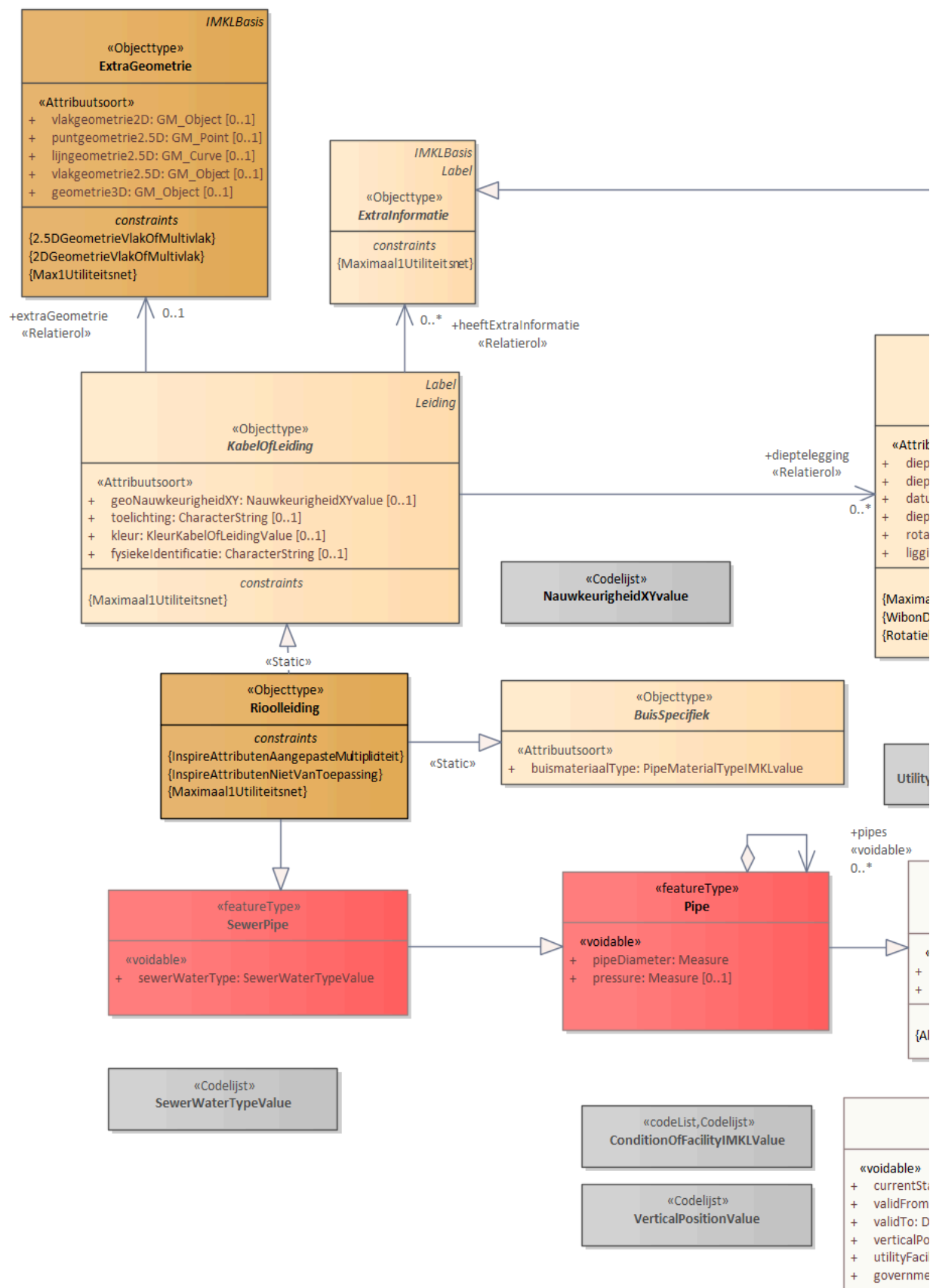
Figuur 22 Rioolleiding
