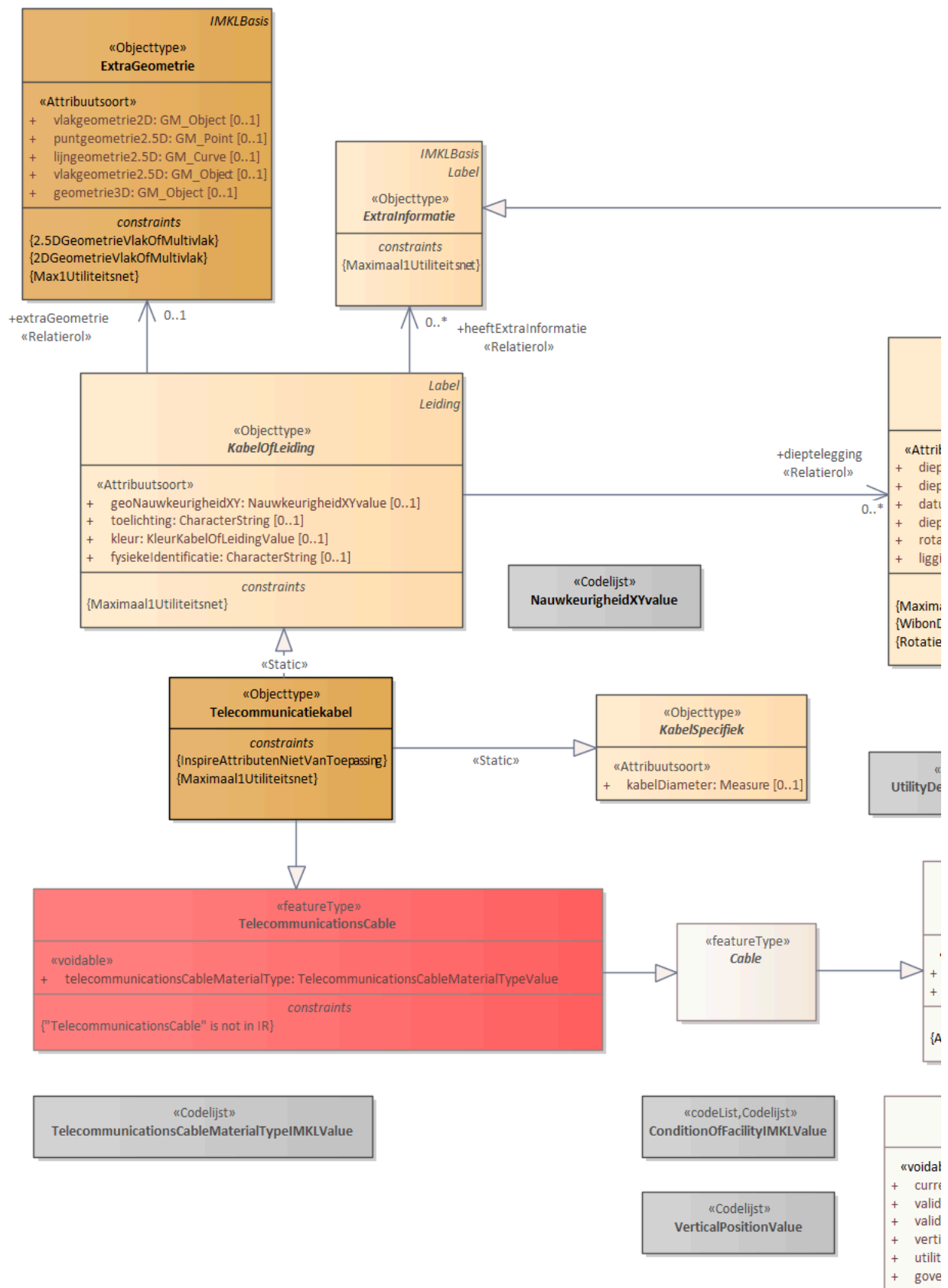
Figuur 20 Telecommunicatiekabel
