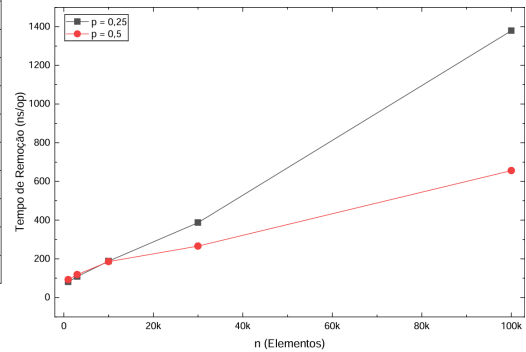
Figura 26: Impacto direto do tempo de busca otimizado na velocidade da operação de exclusão de nós.
