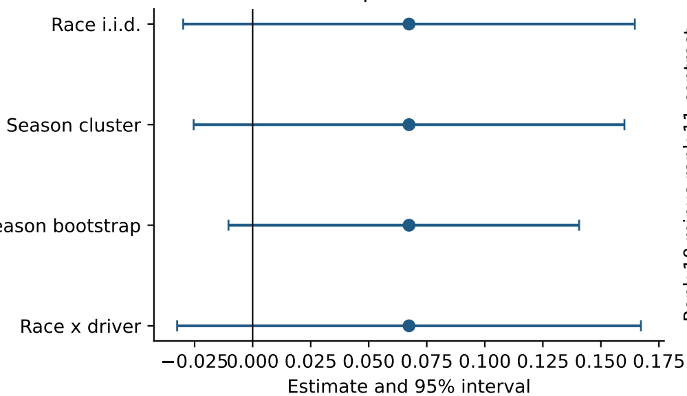
Top-ten finish
