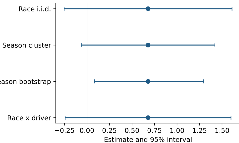
Top-ten finish
