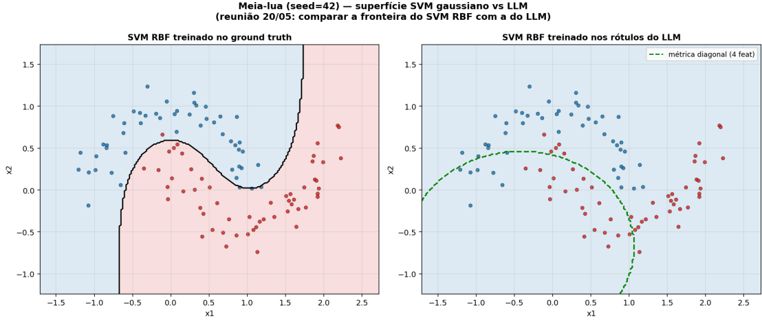
Figura 6: Problema F (meia-lua, seed 42, gpt-4o-mini): superfície de separação do SVM RBF treinado no ground truth (esq.) vs. treinado nos rótulos zero-shot do LLM (dir.). Em ambos os painéis os pontos aparecem nas classes corretas ( ground truth , azul/vermelho): à direita, a lua vermelha inteira cai na região azul, evidenciando que o LLM erra muito mais que o SVM RBF de referência, que não erra nenhum ponto. Nas sementes 123 e 7 o zero-shot colapsa em classe única e o protocolo é abortado.
