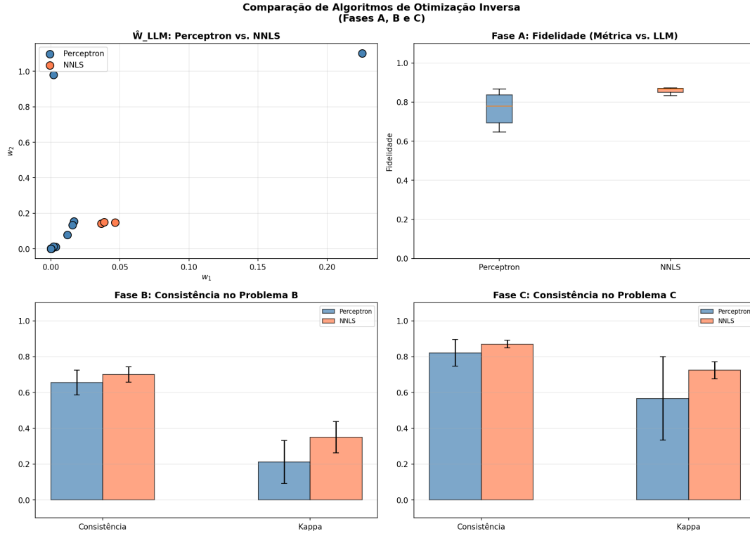
Figura 1: Bloco 1: comparação Perceptron \times NNLS (fidelidade no Problema A, consistência nas Fases nos Problemas B/C e dispersão das direções de \hat{W} estimadas). Os dois estimadores produzem métricas quase colineares (cosseno 0,986).
