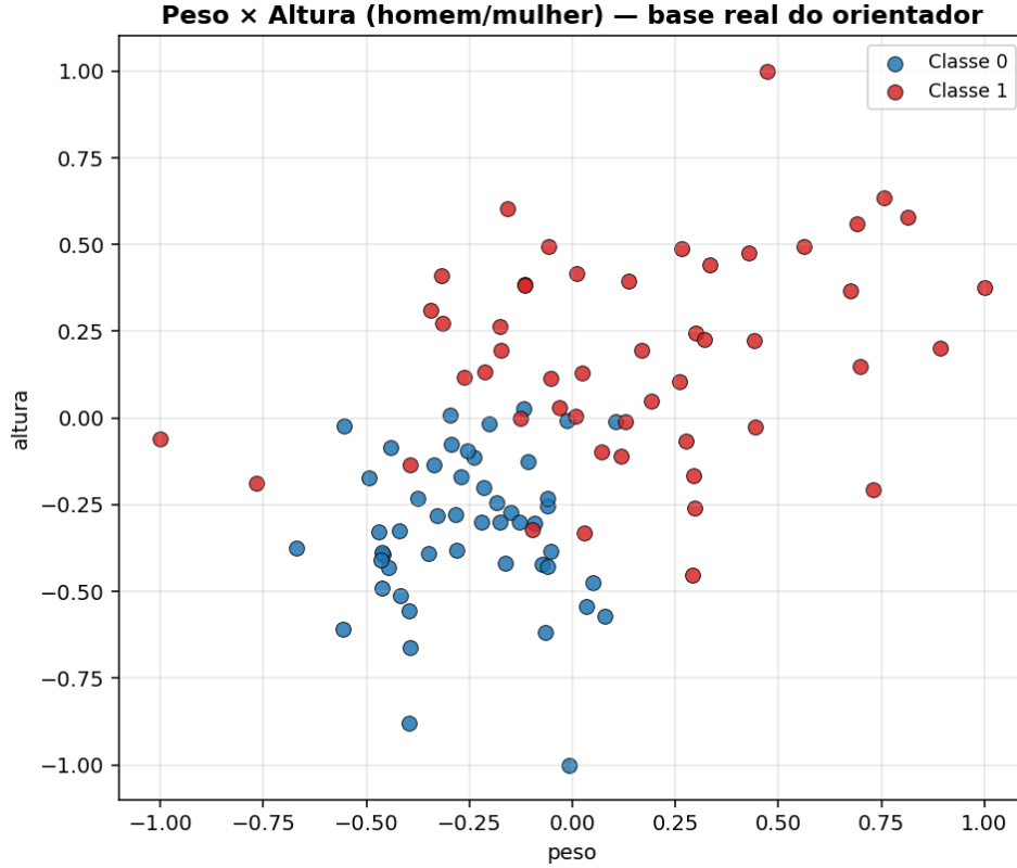
Figura 8: Bloco 3: base real peso \times altura (rótulo homem/mulher) com a fronteira aproximadamente elíptica. A pequena escala ( \approx 70 100 amostras, 70 de treino por semente) motiva o reporte de erros absolutos além das porcentagens.
