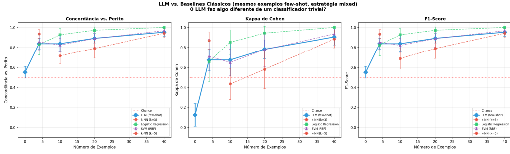
Figura 5: Bloco 2: LLM in-context com aprendizado em contexto vs. baselines clássicas (k-NN, Regressão Logística, SVM-RBF) nos mesmos exemplos few-shot. No regime linear, todos os métodos ficam numa faixa estreita, sem dominância clara.
