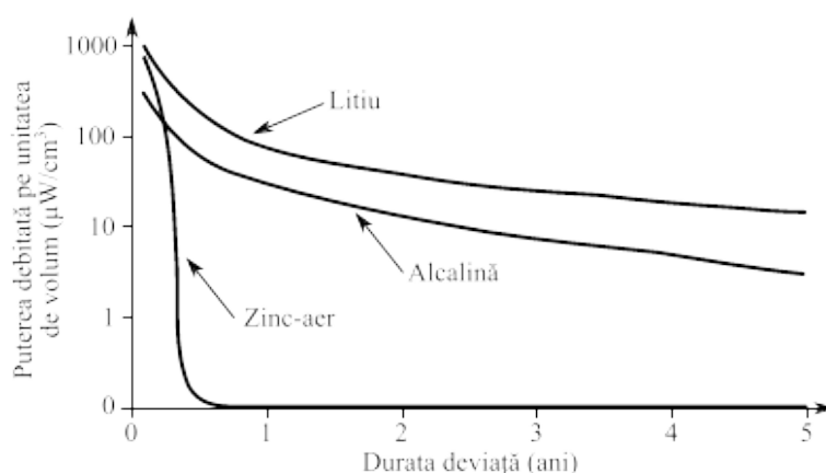
Figura 2.1. Puterea furnizată pe \text{cm}^3 relativă la durata de viață pentru trei tipuri de baterii.
