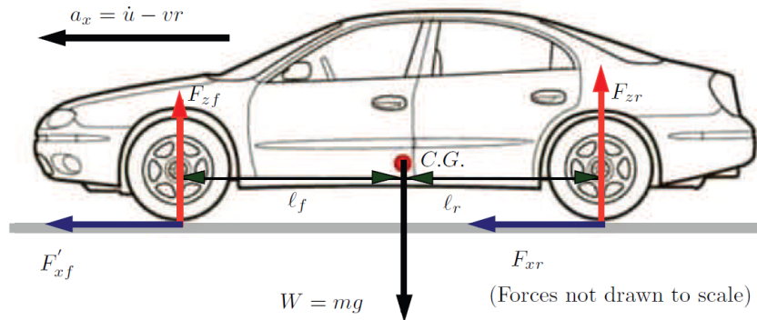
Σχήμα 12: Διάγραμμα ελευθέρου σώματος – διαμήκης μεταφορά βάρους [19].
