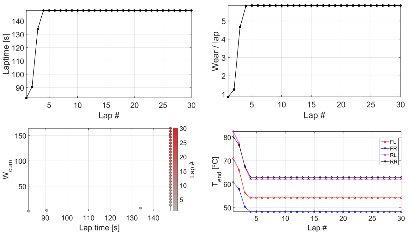
Σχήμα 38: Αποτελέσματα stint 30 γύρων: χρόνος γύρου, φθορά ανά γύρο, σωρευτική φθορά έναντι χρόνου γύρου (χρωματισμός κατά k ), τελικές θερμοκρασίες ανά ελαστικό.
