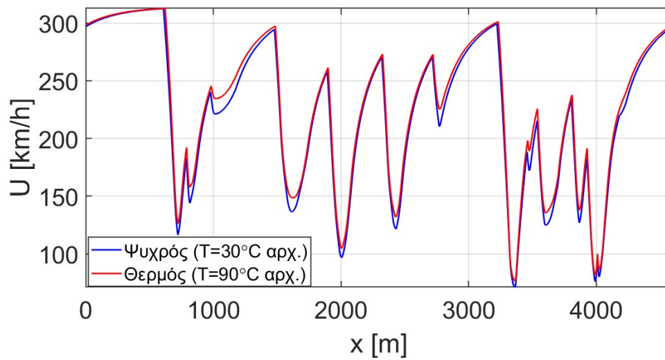
Σχήμα 36: Προφίλ ταχύτητας U(x) για ψυχρό ( 30^\circ\text{C} ) και θερμό ( 90^\circ\text{C} ) γύρο.
