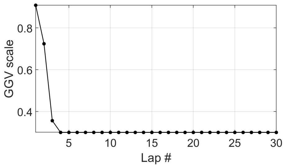
Σχήμα 39: Συντελεστής κλίμακας του φακέλου GGV που χρησιμοποιήθηκε σε κάθε γύρο.
