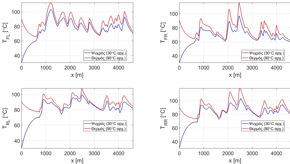
Σχήμα 37: Εξέλιξη θερμοκρασίας T_i(x) ανά ελαστικό για ψυχρό και θερμό γύρο.
