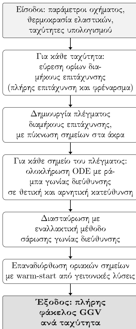
Σχήμα 13: Ροή δημιουργίας διαγράμματος GGV. Το πλέγμα ταχύτητας-διαμήκους επιτάχυνσης σαφώνεται με ολοκλήρωση δυναμικού μοντέλου οχήματος υπό ράμπα γωνίας διεύθυνσης· κάθε σημείο δίνει ένα άνω και ένα κάτω όριο πλευρικής επιτάχυνσης. Ασυγκλίσια και οριακές περιπτώσεις αντιμετωπίζονται μέσω διαδοχικών επιπέδων επίλυσης, ώστε ο τελικός φάκελος GGV να είναι πλήρης και ομαλός. Οι αριθμητικές λεπτομέρειες κάθε βήματος αναλύονται στο κείμενο.
