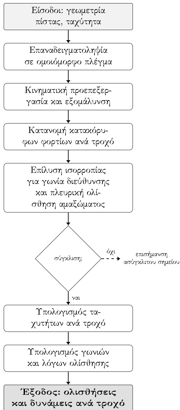
Σχήμα 12: Ροή εκτίμησης ολισθήσεων και δυνάμεων ανά τροχό από δεδομένα πίστας και ταχύτητας. Το ακριβές περιεχόμενο κάθε βήματος (κινηματικές σχέσεις, κριτήριο σύγκλισης, μοντέλο κατανομής φορτίων) περιγράφεται στο κείμενο.
