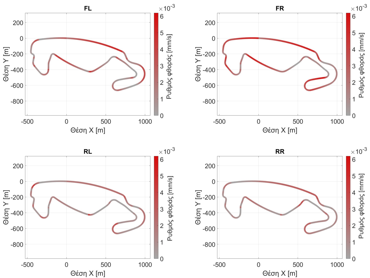
Σχήμα 34: Ρυθμός φθοράς κάθε ελαστικού κατά μήκος της πίστας Circuit de Barcelona - Catalunya .
