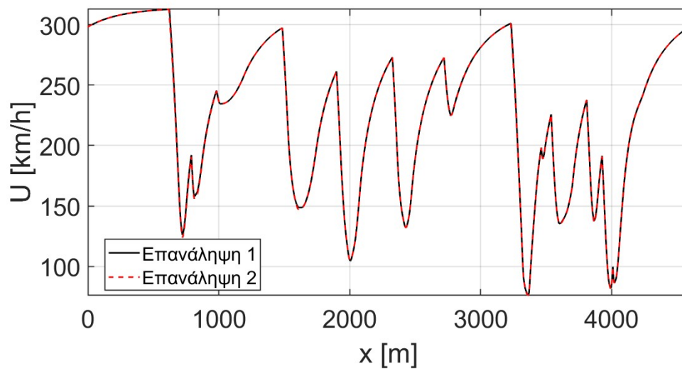
Σχήμα 30: Προφίλ ταχύτητας U(x) για τις δύο διαδοχικές επαναλήψεις.
