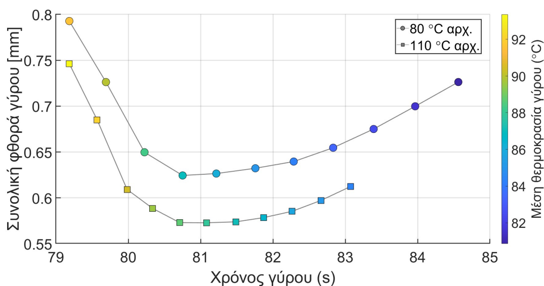
Σχήμα 36: Διάγραμμα χρόνου – συνολικής φθοράς
