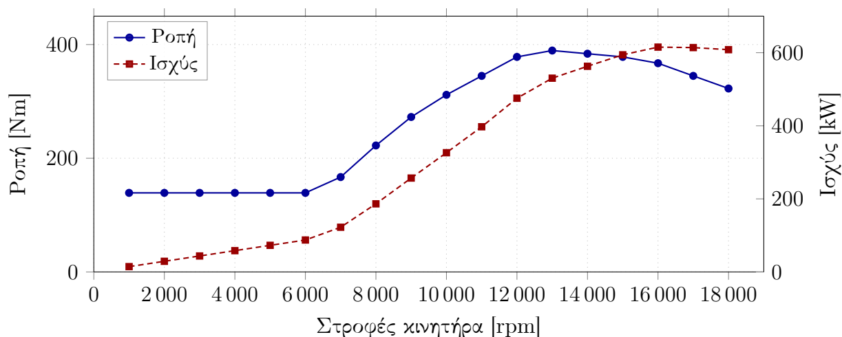
Σχήμα 31: Καμπύλη ροπής κινητήρα.
