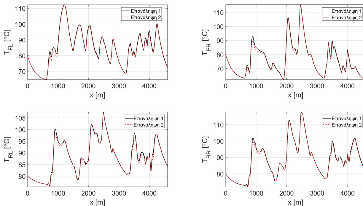
Σχήμα 29: Σύγκριση T_i(x) ανά ελαστικό ανάμεσα στην πρώτη (σταθερές συνθήκες) και στη δεύτερη επανάληψη (μεταβαλλόμενες συνθήκες).
