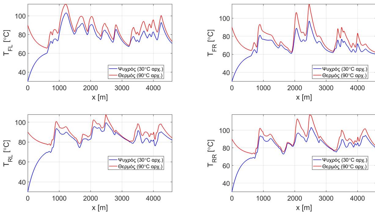
Σχήμα 38: Εξέλιξη θερμοκρασίας T_i(x) ανά ελαστικό για ψυχρό και θερμό γύρο.
