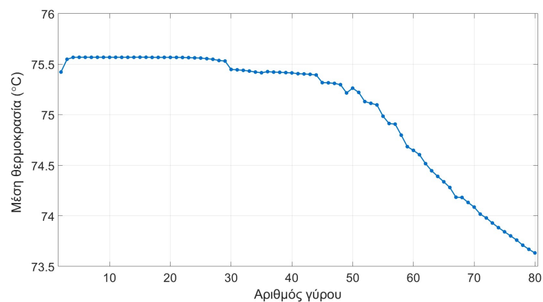
Σχήμα 41: Μέση θερμοκρασία ελαστικών συναρτήσει του αριθμού των γύρων ( Circuit de Barcelona-Catalunya )
