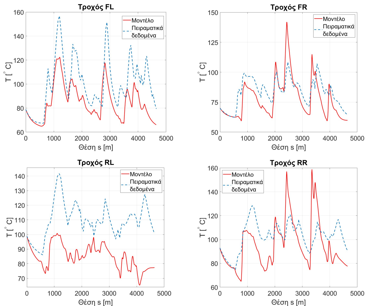
Σχήμα 32: Σύγκριση θερμοκρασίας μοντέλου με πειραματική σε γύρο της πίστας Circuit de Barcelona - Catalunya
