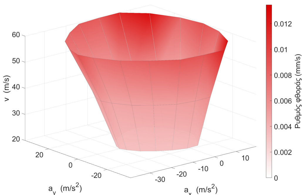
Σχήμα 35: Διάγραμμα επιδόσεων στα T_{\text{tyre}} = 110^{\circ}\text{C} , με χρώμα τον συνολικό ρυθμό φθοράς και των τεσσάρων ελαστικών σε κάθε σημείο πλέγματος.
