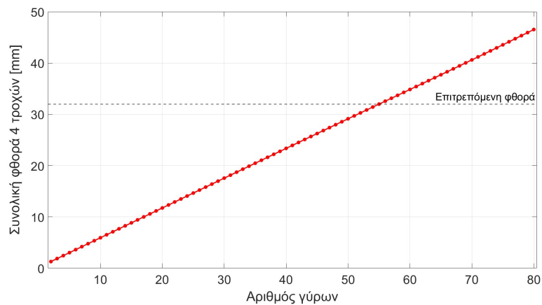
Σχήμα 40: Συνολική φθορά συναρτήσει του αριθμού των γύρων ( Circuit de Barcelona-Catalunya )
